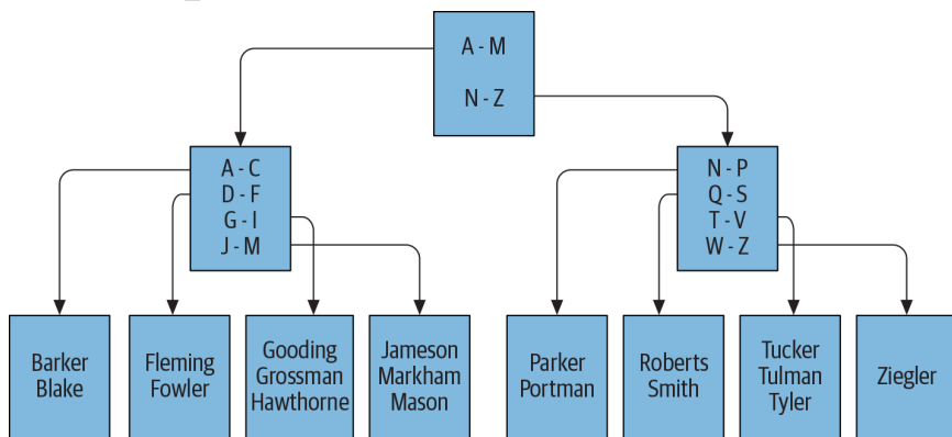
Рис. 13.1. Пример сбалансированного дерева B-tree
