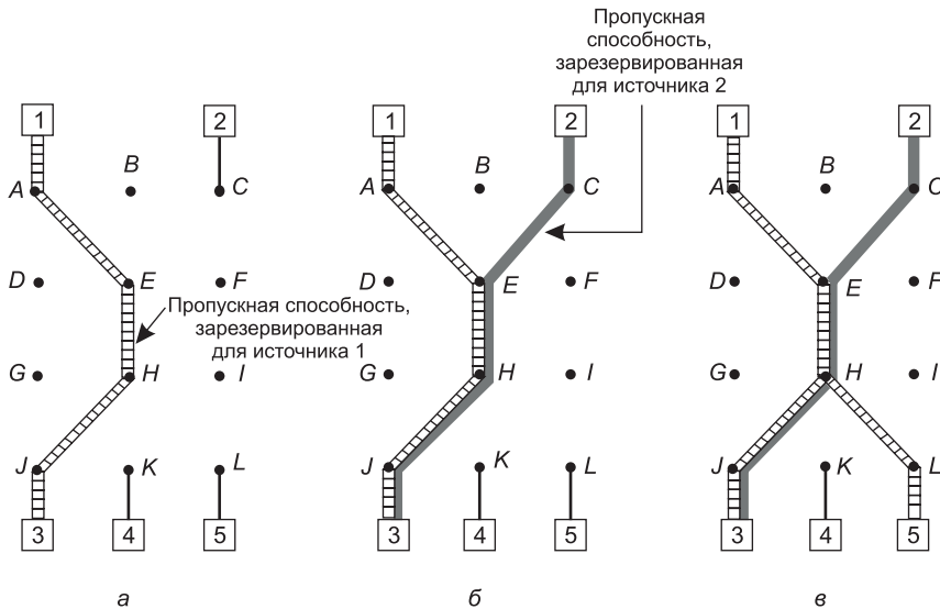
Рис. 5.31. Пример резервирования: а — хост 3 запрашивает канал к хосту 1; б — затем хост 3 запрашивает второй канал к хосту 2; в — хост 5 запрашивает канал к хосту 1
