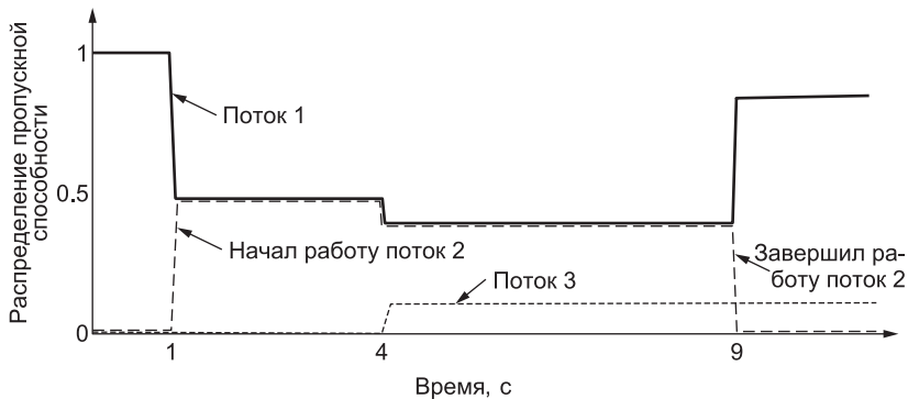
Рис. 6.18. Изменение распределения пропускной способности с течением времени
