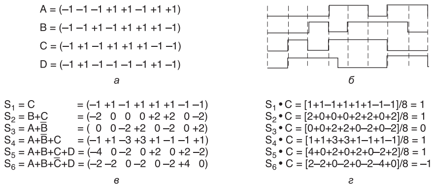
Рис. 2.24. Последовательности: а — двоичные элементарные последовательности для четырех станций; б — биполярные элементарные двоичные последовательности; в — шесть примеров передачи; г — восстановление сигнала станции C
