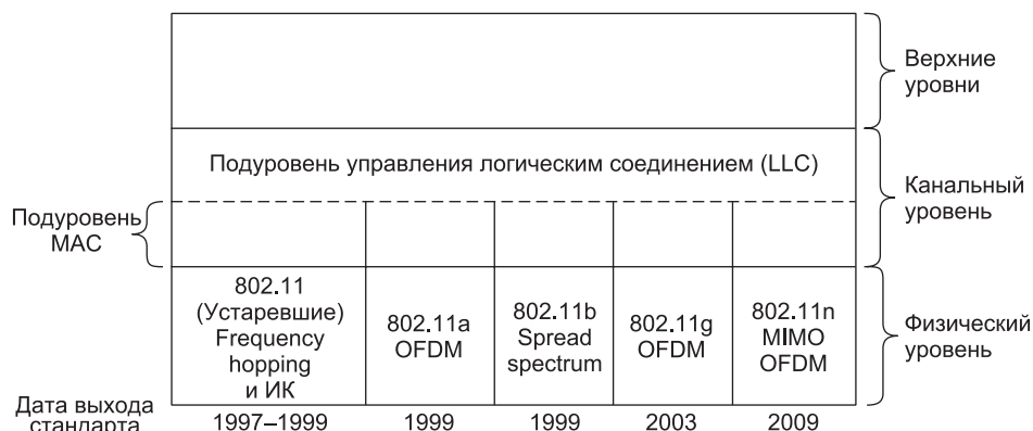
Рис. 4.21. Часть стека протоколов 802.11
