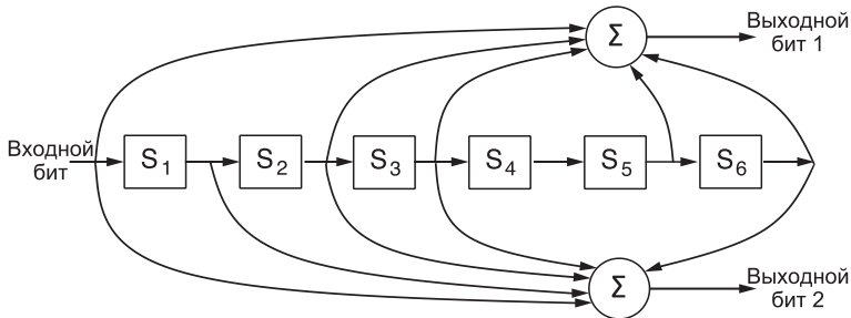
Рис. 3.7. Двоичный сверточный код NASA применяется в сетях 802.11
