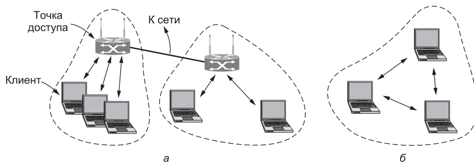
Рис. 4.20. Архитектура сети стандарта 802.11: а — инфраструктурный режим; б — произвольный режим
