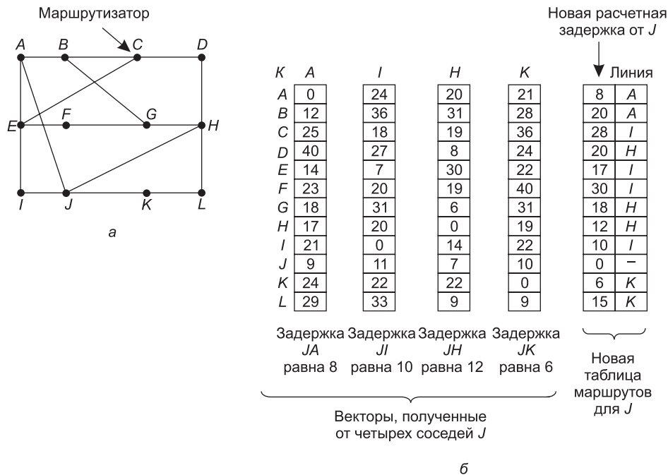
Рис. 5.7. Сеть (а); полученные от A , I , H и K векторы и новая таблица маршрутов для J (б)
