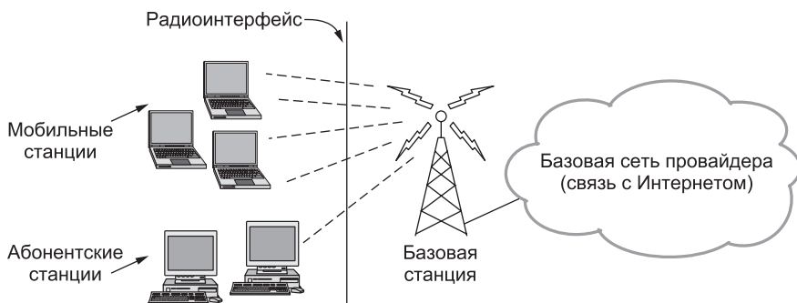
Рис. 4.27. Архитектура стандарта 802.16
