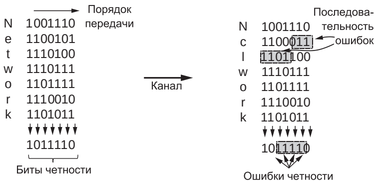
Рис. 3.8. Чередование битов четности для обнаружения последовательностей ошибок
