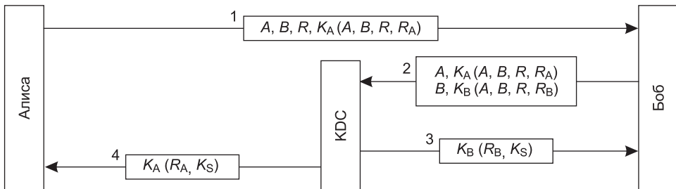
Рис. 8.37. Протокол аутентификации Отуэя—Риса (слегка упрощенный)
