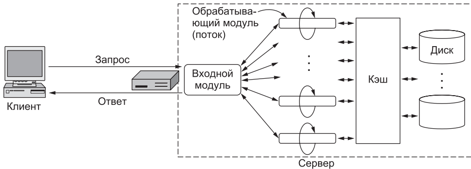
Рис. 7.9. Многопоточный веб-сервер с входным и обрабатывающими модулями
