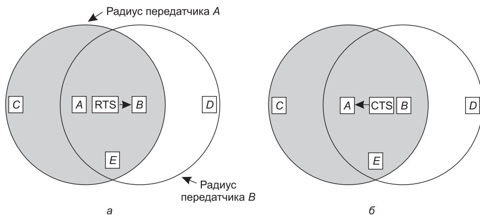
Рис. 4.12. Протокол MACA: а — станция A посылает кадр RTS станции B ; б — станция B отвечает кадром CTS станции A
