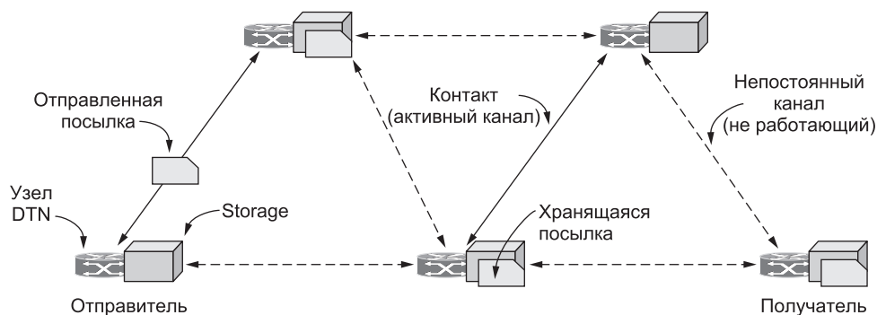
Рис. 6.50. Архитектура DTN
