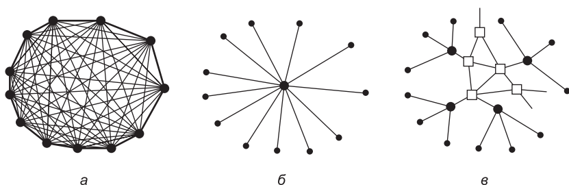
Рис. 2.25. Сеть «каждый с каждым» (а); централизованный коммутатор (б); двухуровневая иерархия (в)
