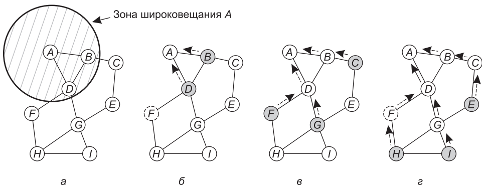
Рис. 5.18. Произвольная сеть: а — зона широковещания A ; б — состояние после получения его узлами B и D ; в — состояние после получения его узлами C , F и G ; г — состояние после получения его узлами E , H и I . Затененными кружочками обозначены новые получатели. Пунктиром показаны возможные обратные маршруты. Сплошными линиями показан построенный маршрут
