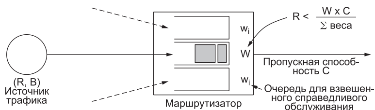
Рис. 5.29. Гарантии пропускной способности и задержки с использованием маркерных ведер и взвешенного справедливого обслуживания
