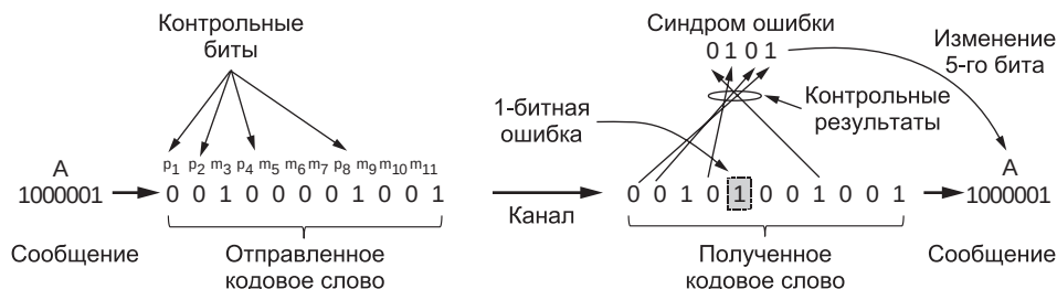
Рис. 3.6. Пример кода Хэмминга (11,7), исправляющего однобитную ошибку
