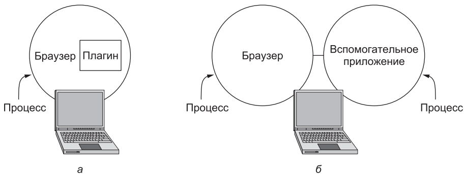
Рис. 7.8. Браузер с подключаемым модулем (а); вспомогательное приложение (б)
