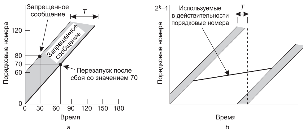
Рис. 6.7. Сегменты не могут заходить в запретную зону (а); проблема ресинхронизации (б)
