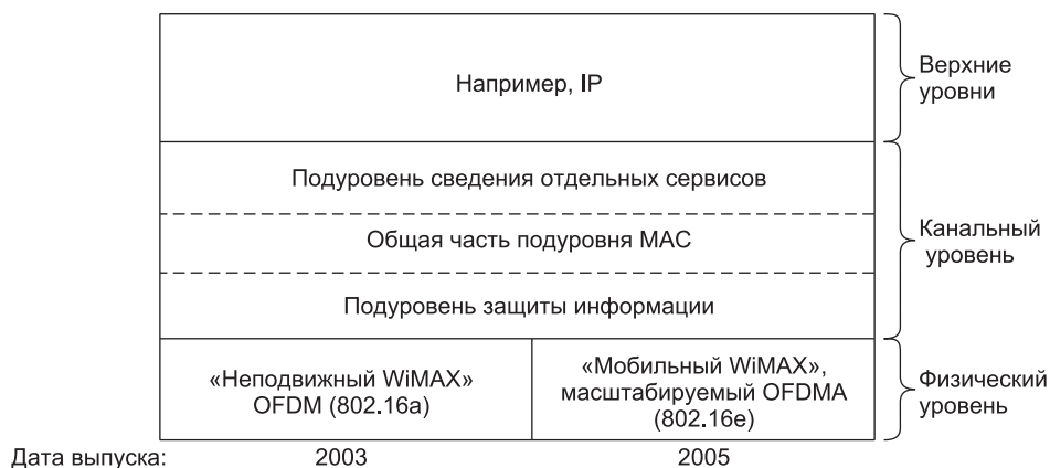
Рис. 4.28. Стек протоколов 802.16
