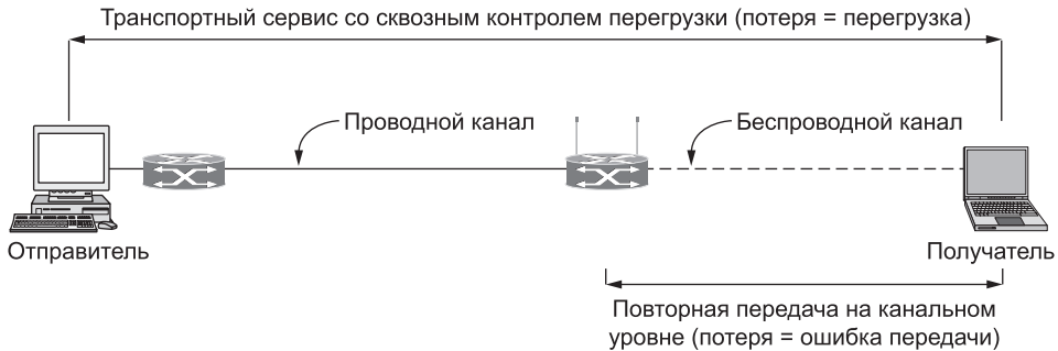
Рис. 6.22. Контроль перегрузки для пути, содержащего беспроводной канал
