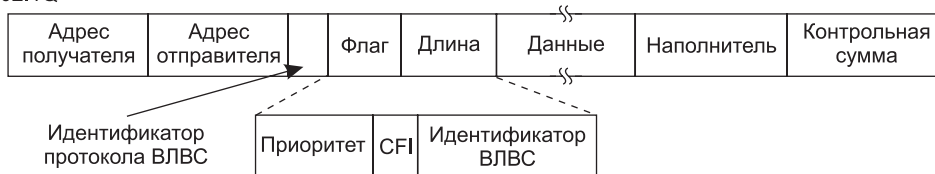
Рис. 4.46. Форматы кадров Ethernet-стандартов 802.3 и 802.1Q
