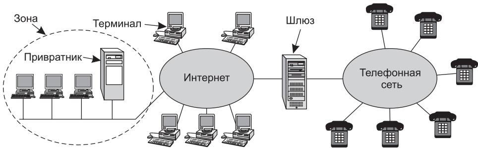
Рис. 7.33. Модель архитектуры H.323 для интернет-телефонии
