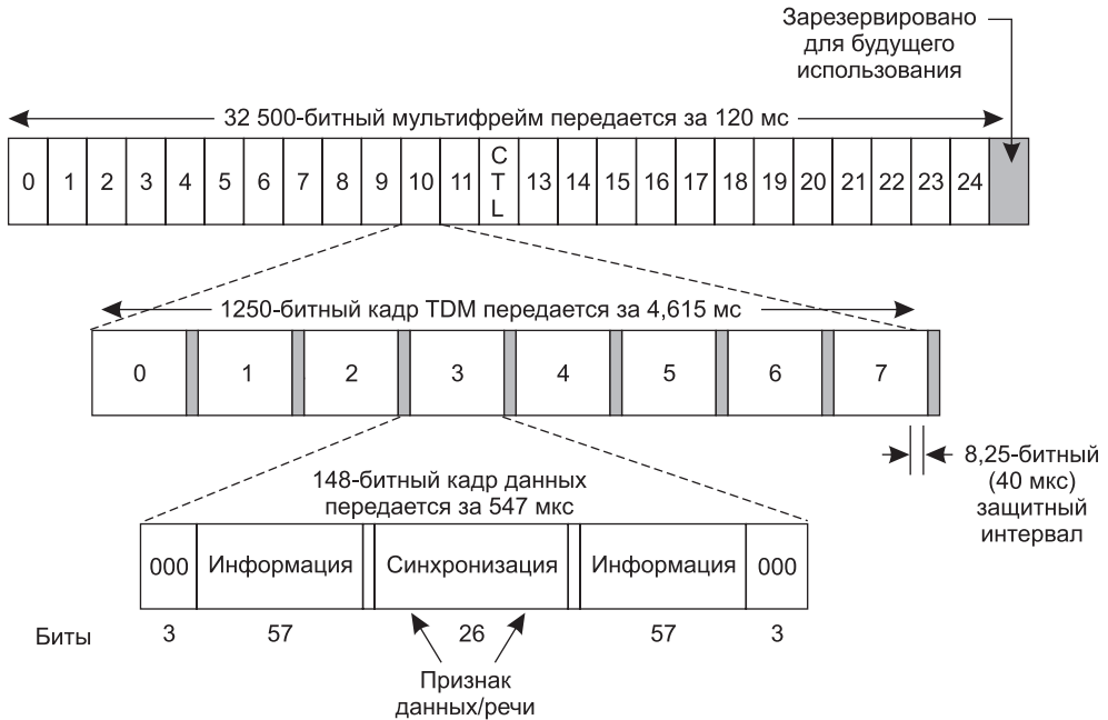
Рис. 2.42. Часть иерархической структуры кадров GSM
