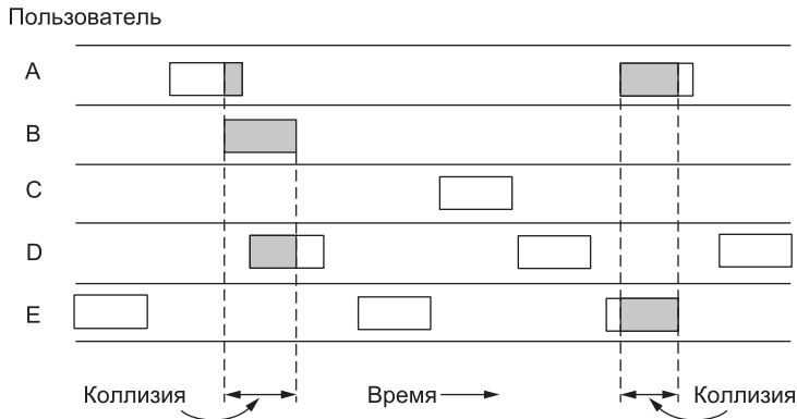
Рис. 4.1. В чистой системе ALOHA кадры передаются в абсолютно произвольное время
