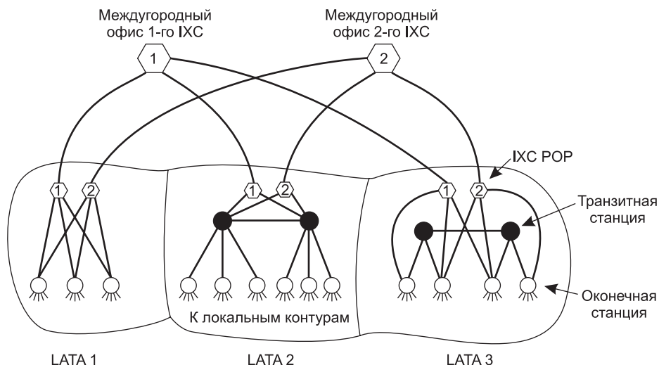
Рис. 2.27. Взаимоотношение между LATA, LEC и IXC. Кружками обозначены коммутаторы ЛЕС. Шестиугольники принадлежат IXC, номер которых указан внутри
