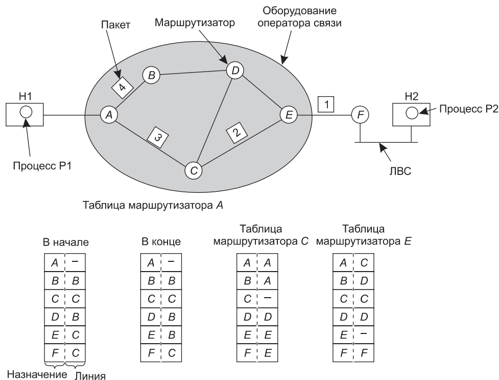
Рис. 5.2. Маршрутизация внутри дейтаграммной подсети
