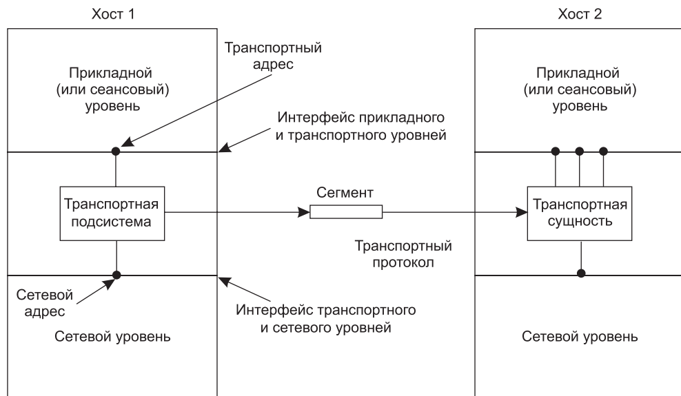
Рис. 6.1. Сетевой, транспортный и прикладной уровни
