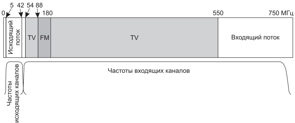
Рис. 2.46. Распределение частот в типичной системе кабельного телевидения, используемой для доступа в Интернет
