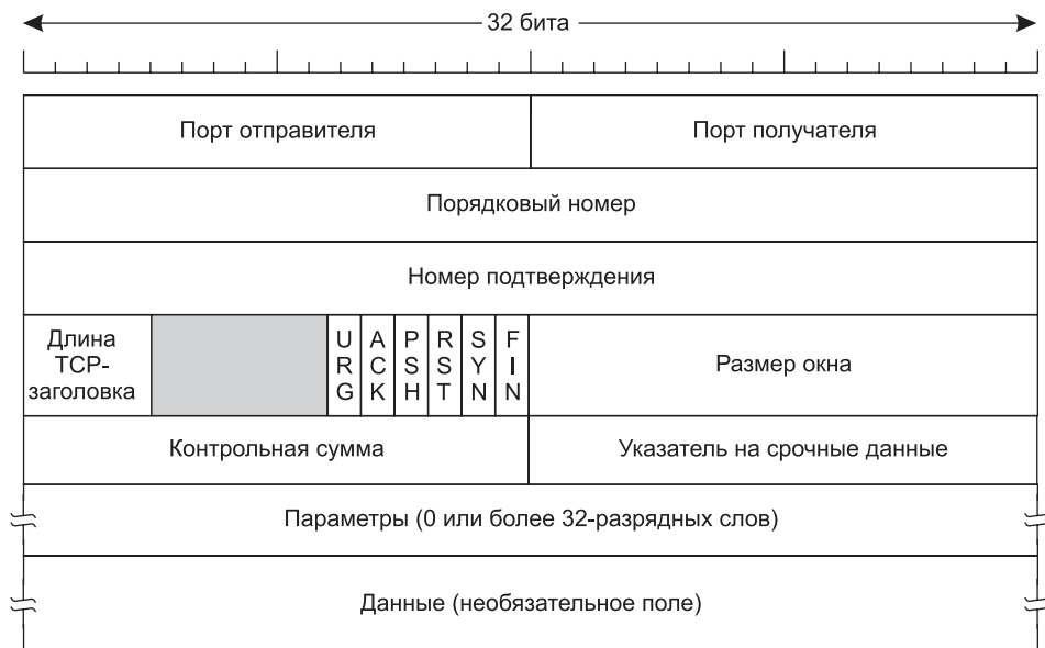
Рис. 6.31. Заголовок TCP
