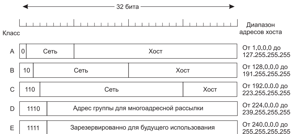
Рис. 5.46. Форматы IP-адреса
