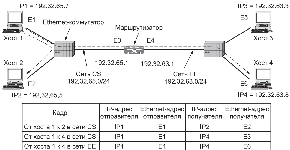
Рис. 5.52. Две коммутируемые ЛВС Ethernet, соединенные маршрутизатором
