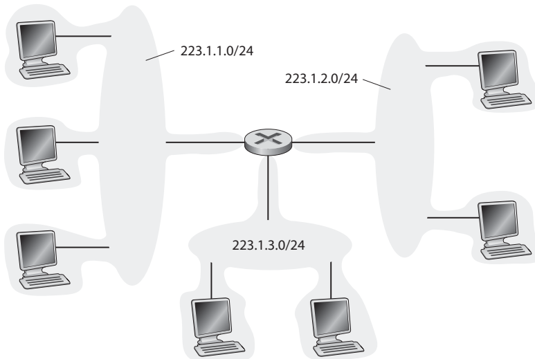
Рис. 4.16. Адреса подсетей
