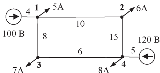
Рис. 70. Схема сети
