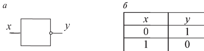
Рис. 14. Элемент НЕ: а — условное изображение; б — таблица состояний
