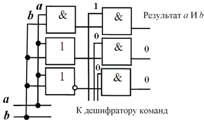
Рис. 26. Работа логического устройства
