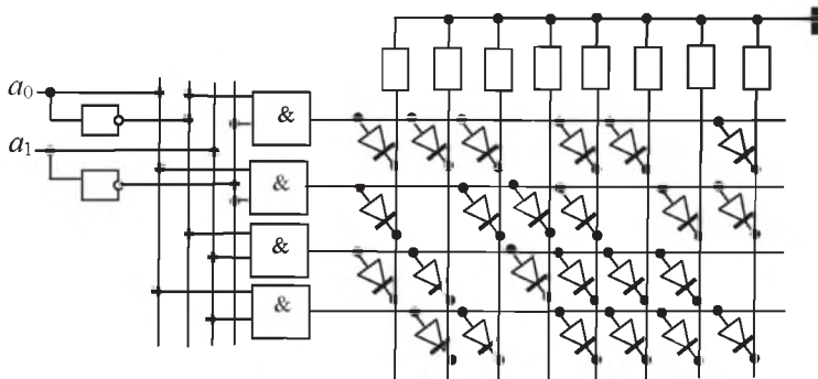
Рис. 31. ROM 4 \times 8
