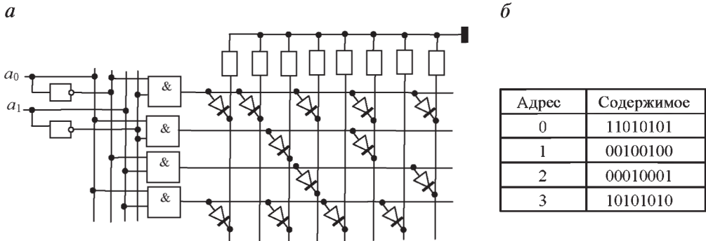
Рис. 30. Масочная ROM 4 \times 8 :
