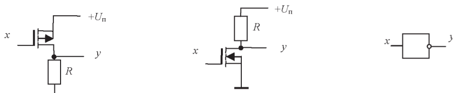
Рис. 21. Инвертор на полевых транзисторах:
