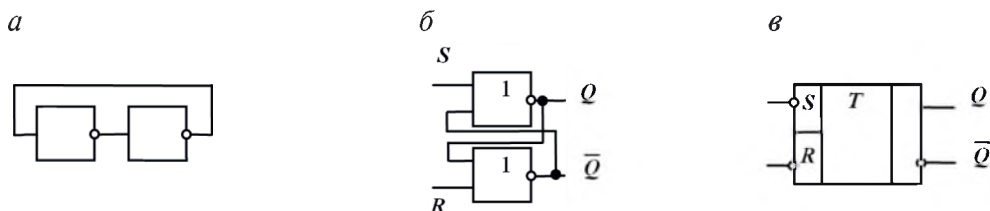
Рис. 27. Асинхронный RS -триггер:
