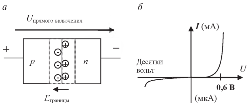
Рис. 12. pn -переход:
