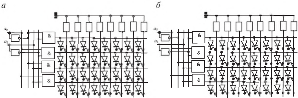
Рис. 33. Память PROM :
