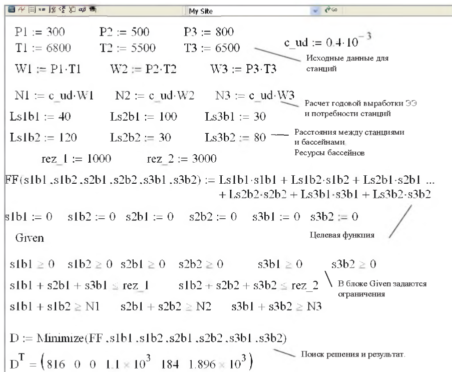
Рис. 92. Транспортная задача
