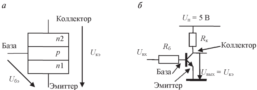
Рис. 13. Биполярный p\bar{n}n -транзистор: а — структурная схема; б — биполярный ключ
