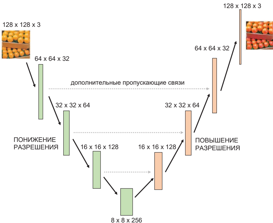
Рис. 5.6. Архитектура U-Net
