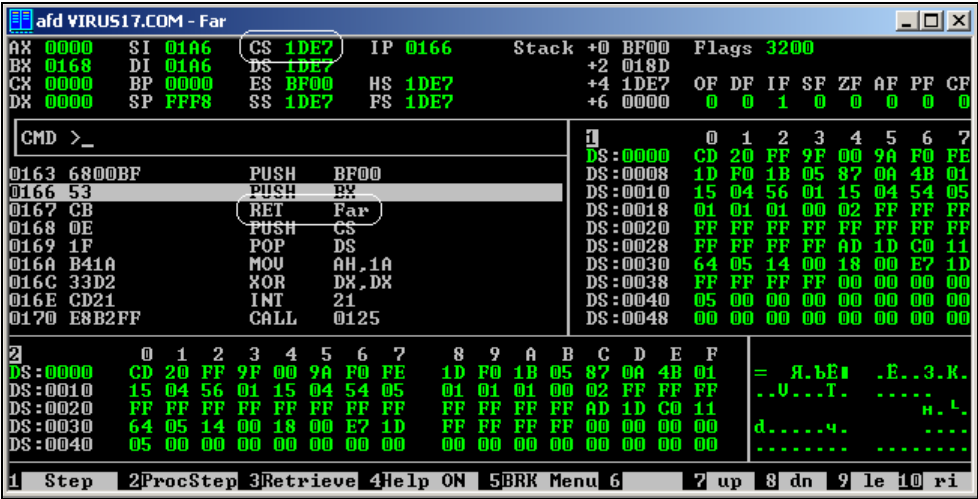
Рис. 17.4. Пока еще в начальном сегменте
