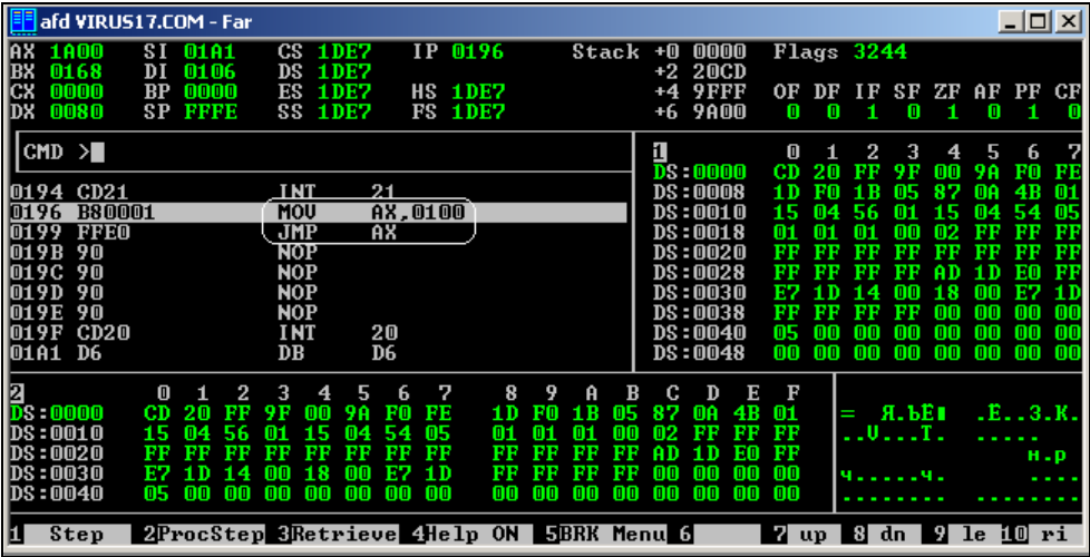
Рис. 17.6. Подготовка к переходу на адрес 100h
