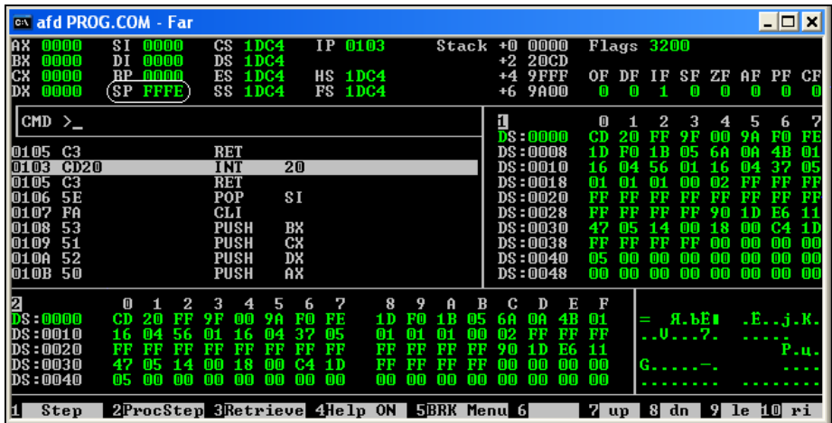
Рис. 6.3. Процедура отработала. Стек выровнен
