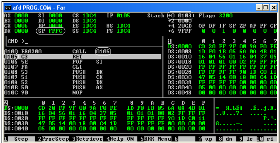
Рис. 6.2. Вызов процедуры с занесением в стек адреса возврата из нее
