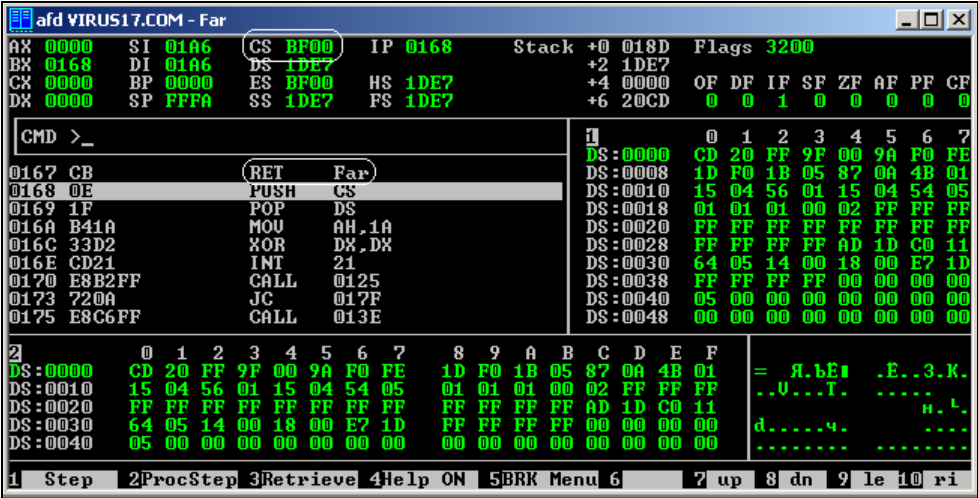
Рис. 17.5. Уже в новом сегменте кода
