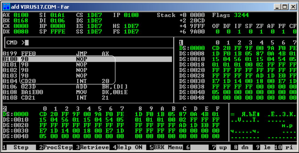
Рис. 17.7. Вот что в конце работы вируса находится по стартовому адресу 100h
