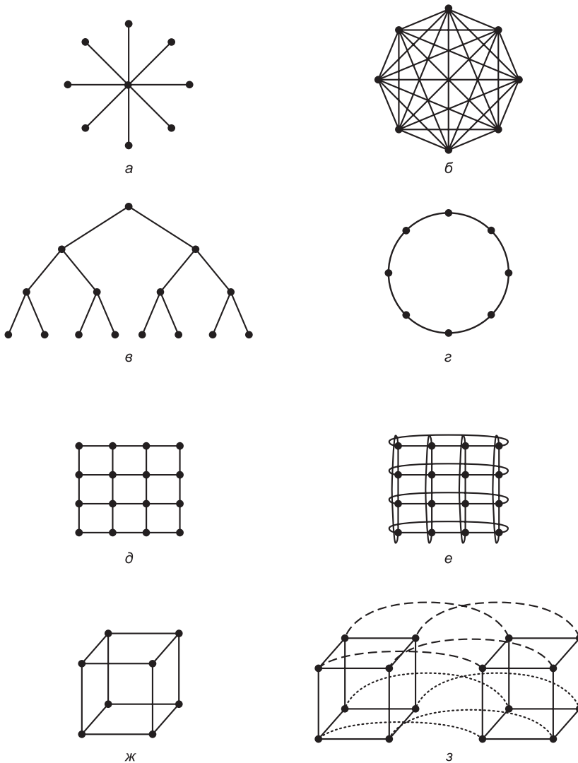
Рис. 8.33. Различные топологии. Жирные точки соответствуют коммутаторам.
