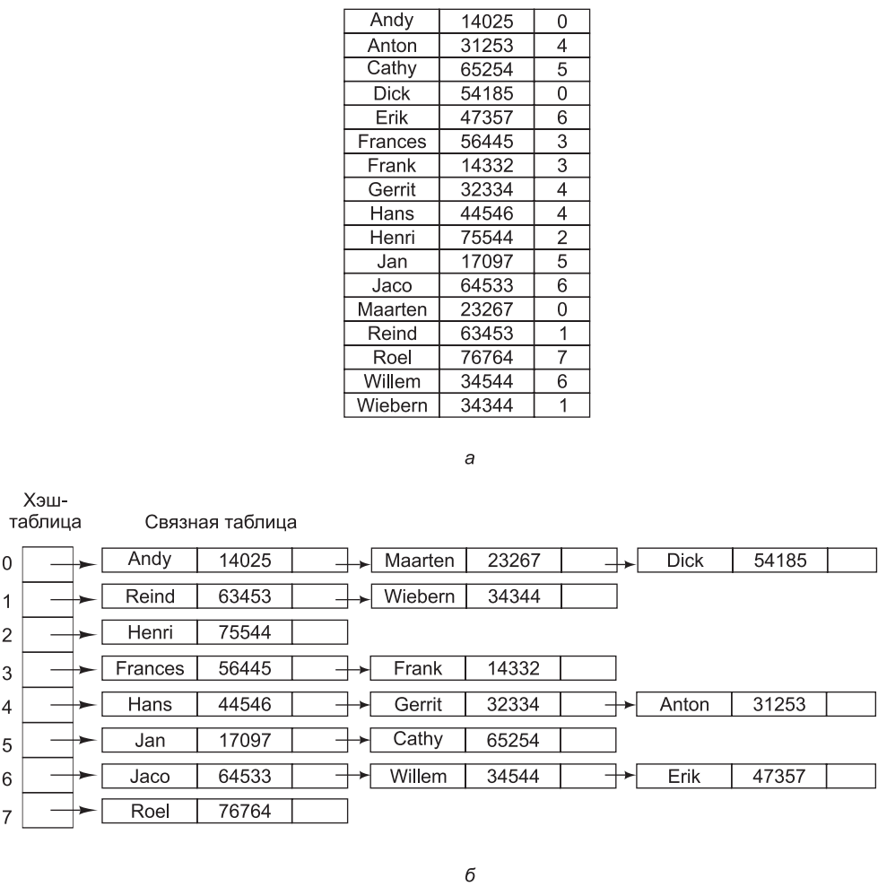
Рис. 7.1. Хеширование: символические имена, значения и хеш-коды, образованные от символических имен (а); хэш-таблица из 8 элементов со связным списком символических имен и значений (б)
