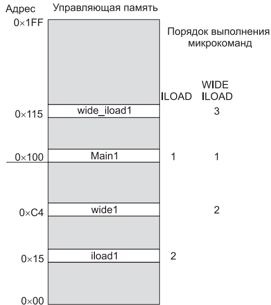
Рис. 4.15. Начало последовательности микрокоманд для команд ILOAD и WIDE ILOAD. Адреса приводятся в качестве примера
