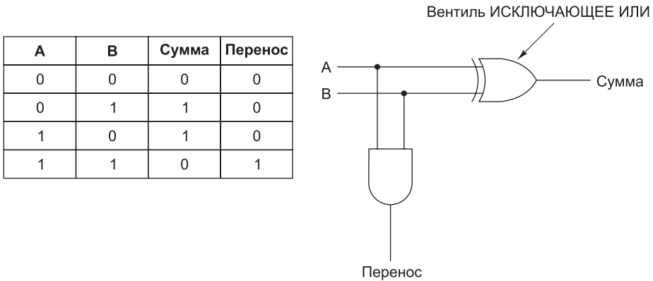
Рис. 3.15. Таблица истинности для сложения одnorазрядных чисел (а); схема полусумматора (б)
