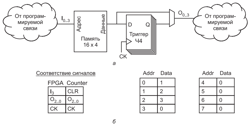
Рис. 3.31. Таблица преобразования FPGA (а); конфигурация LUT для создания 3-разрядного счетчика со сбросом (б)
