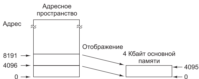
Рис. 6.2. Виртуальные адреса памяти с 4096 по 8191 отображаются на адреса основной памяти с 0 по 4095
