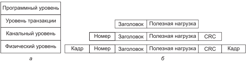
Рис. 3.53. Стек протоколов PCI Express (а); формат пакета (б)
