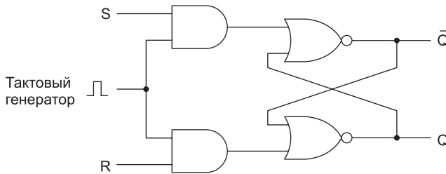
Рис. 3.21. Синхронная SR-защелка
