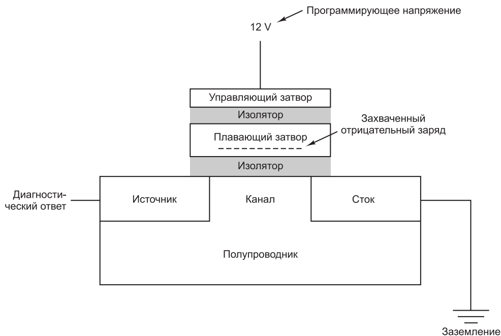
Рис. 2.20. Ячейка флэш-памяти
