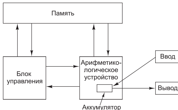
Рис. 1.4. Схема фон-неймановской вычислительной машины
