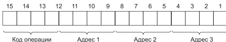
Рис. 5.7. Команда с 4-разрядным кодом операции и тремя 4-разрядными адресными полями
