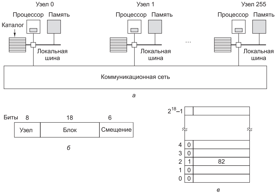
Рис. 8.29. Микропроцессор на основе каталога, содержащий 256 узлов (а); разбиение 32-разрядного адреса памяти на поля (б); каталог в узле 36 (в)
