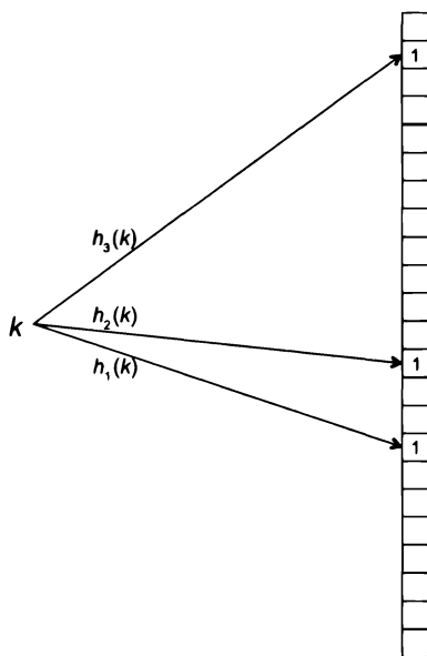
Рис. 12.5. Вставка нового ключа k в фильтр Блума устанавливает биты в позиции h_1(k), \dots, h_m(k) равными 1
