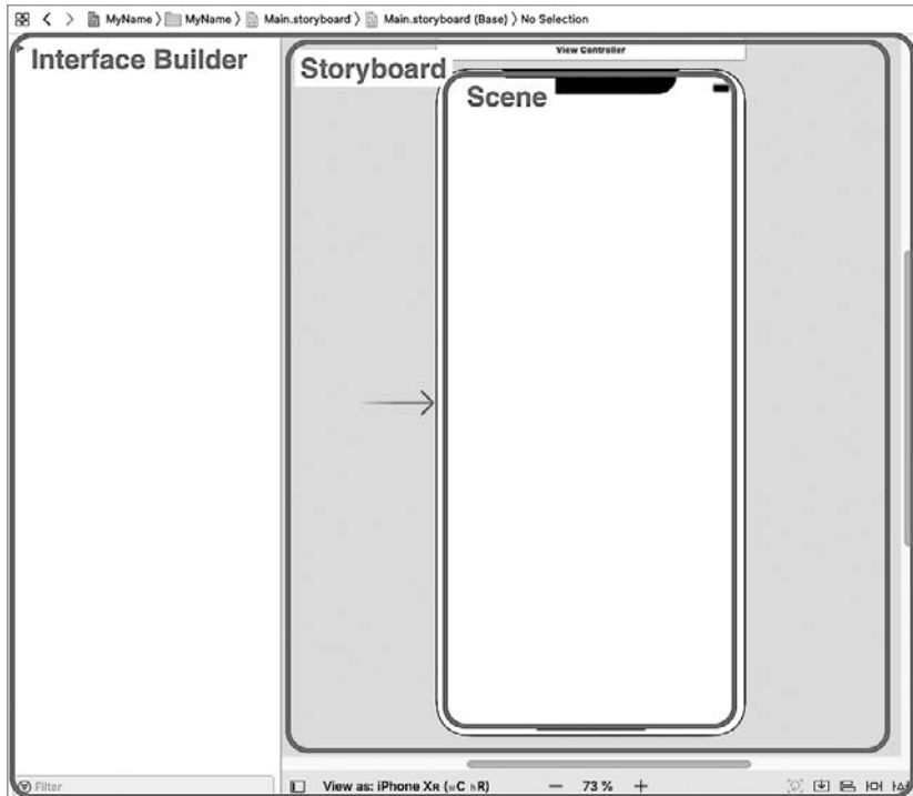
Рис. 38.3. Редактор интерфейса
