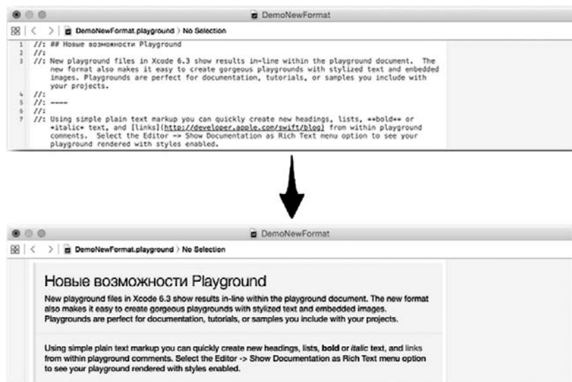
Рис. 1.10. Форматированный комментарий
