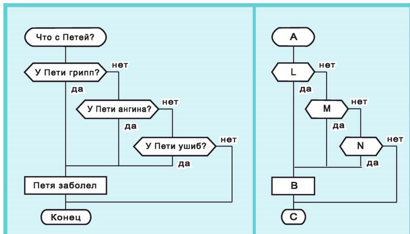
Рис. 110. Примеры алгоритмов с операцией «ИЛИ»
