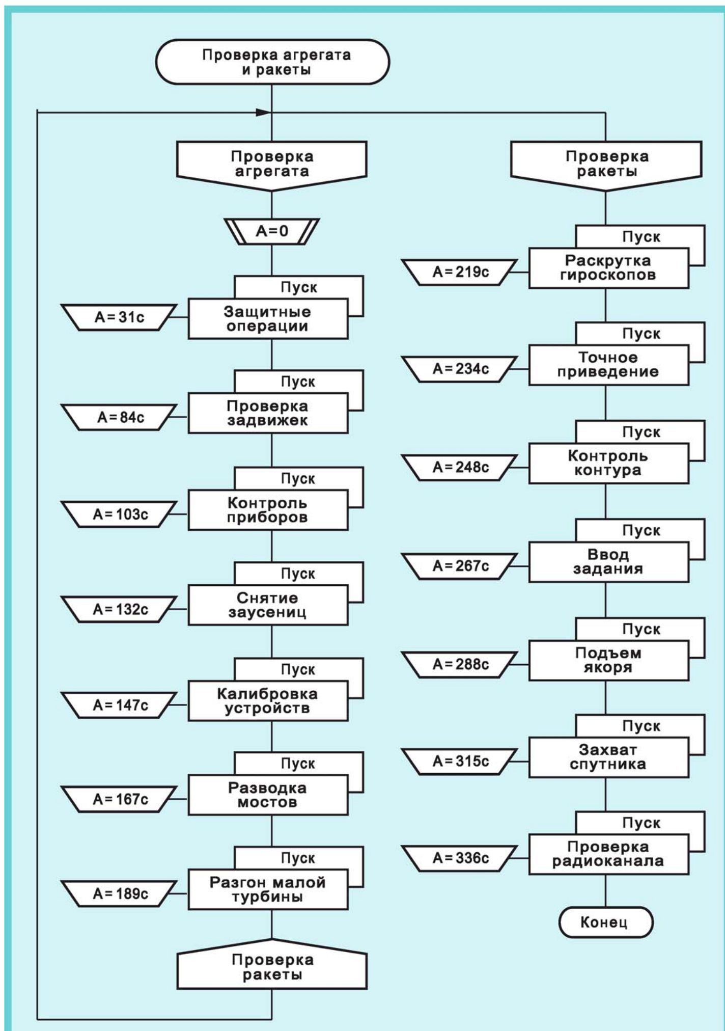
Рис. 149. Алгоритм с параллельными процессами «Проверка агрегата и ракеты»
