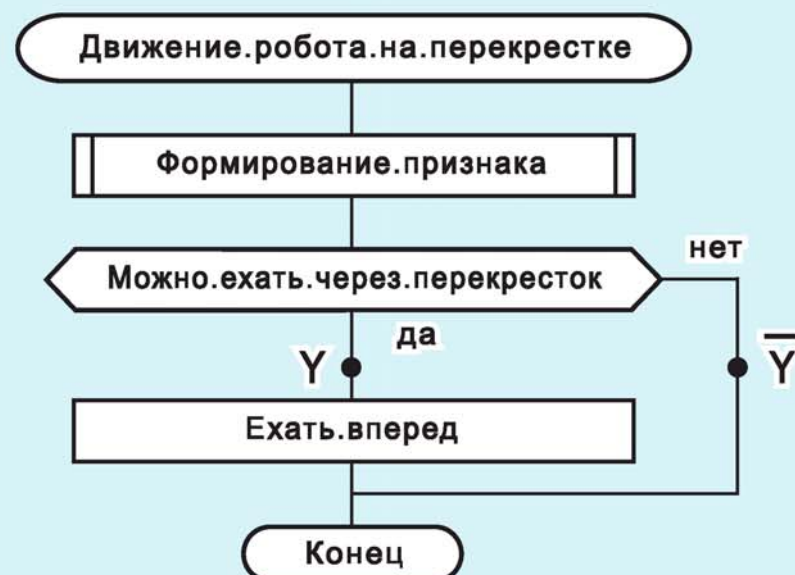
Рис. 136. Добавляем процедуру «Формирование.признака», которая создает признак «Можно.ехать.через.перекресток»
