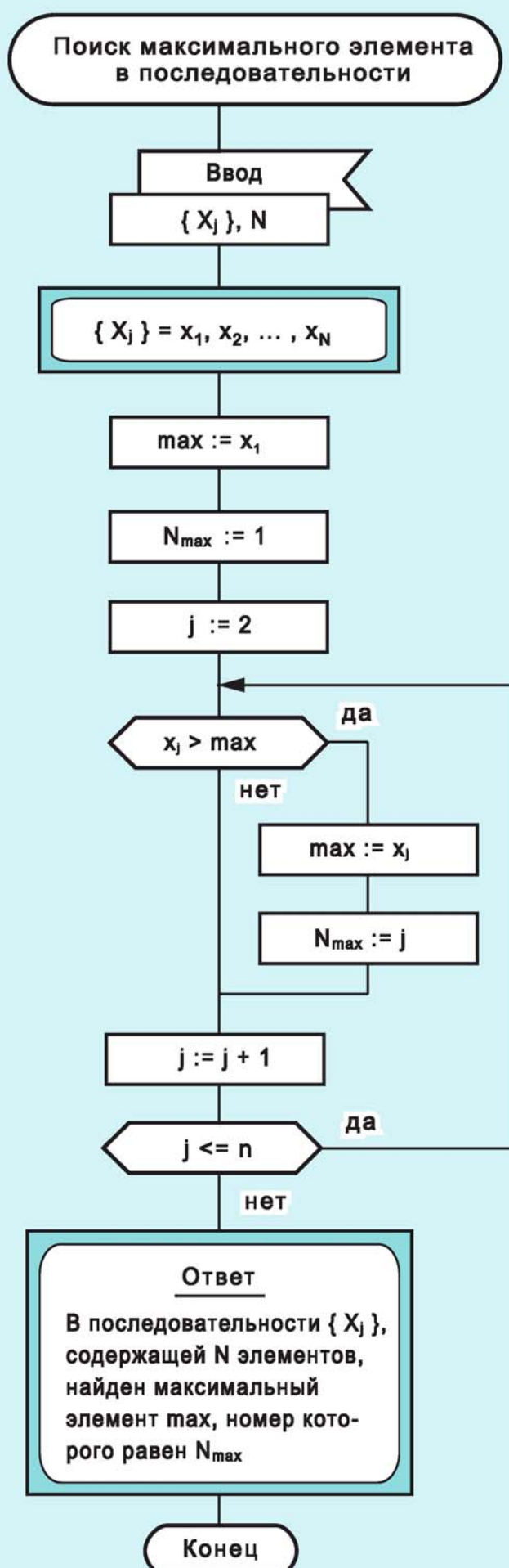
Рис. 215. Поиск максимального элемента в последовательности
