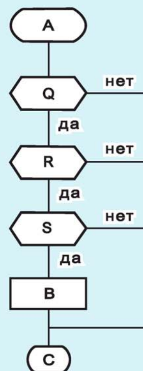
Рис. 105. Примеры алгоритмов с операцией «И»
