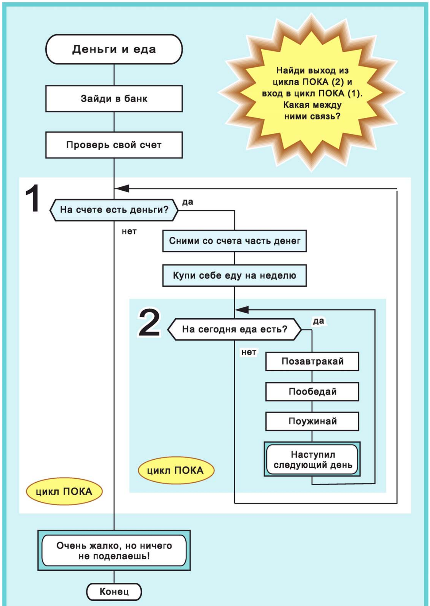
Рис. 98. Деньги и еда. Цикл ПОКА (2) внутри цикла ПОКА (1)
