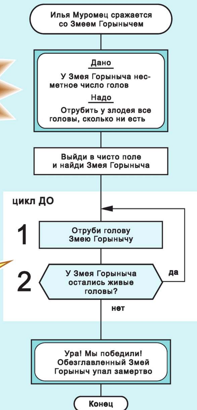
Рис. 77. Хороший (короткий) алгоритм. А почему он короткий? Потому что в нем есть ЦИКЛ. Циклический алгоритм позволяет отрубить любое число голов. При этом нужна всего одна команда «Отруби голову».
