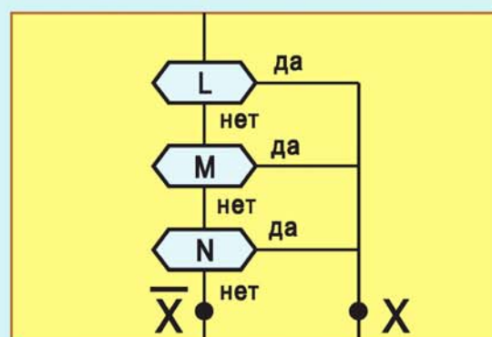
Рис. 122. Стандартный и нестандартный вид логических схем «И», «ИЛИ» для трех логических переменных
