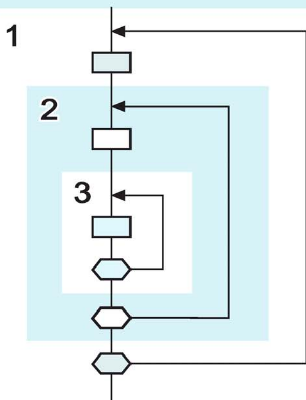
Рис. 101. Цикл ДО (3) внутри цикла ДО (2) внутри цикла ДО (1)
