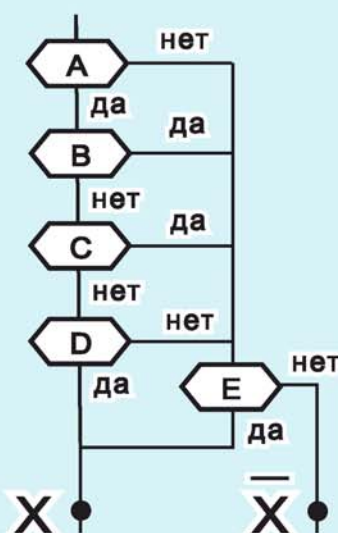
Рис. 125. Какую логическую функцию вычисляют эти схемы?
