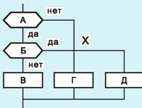
Рис. 63. Плохая схема. Есть пересечение в точке X
