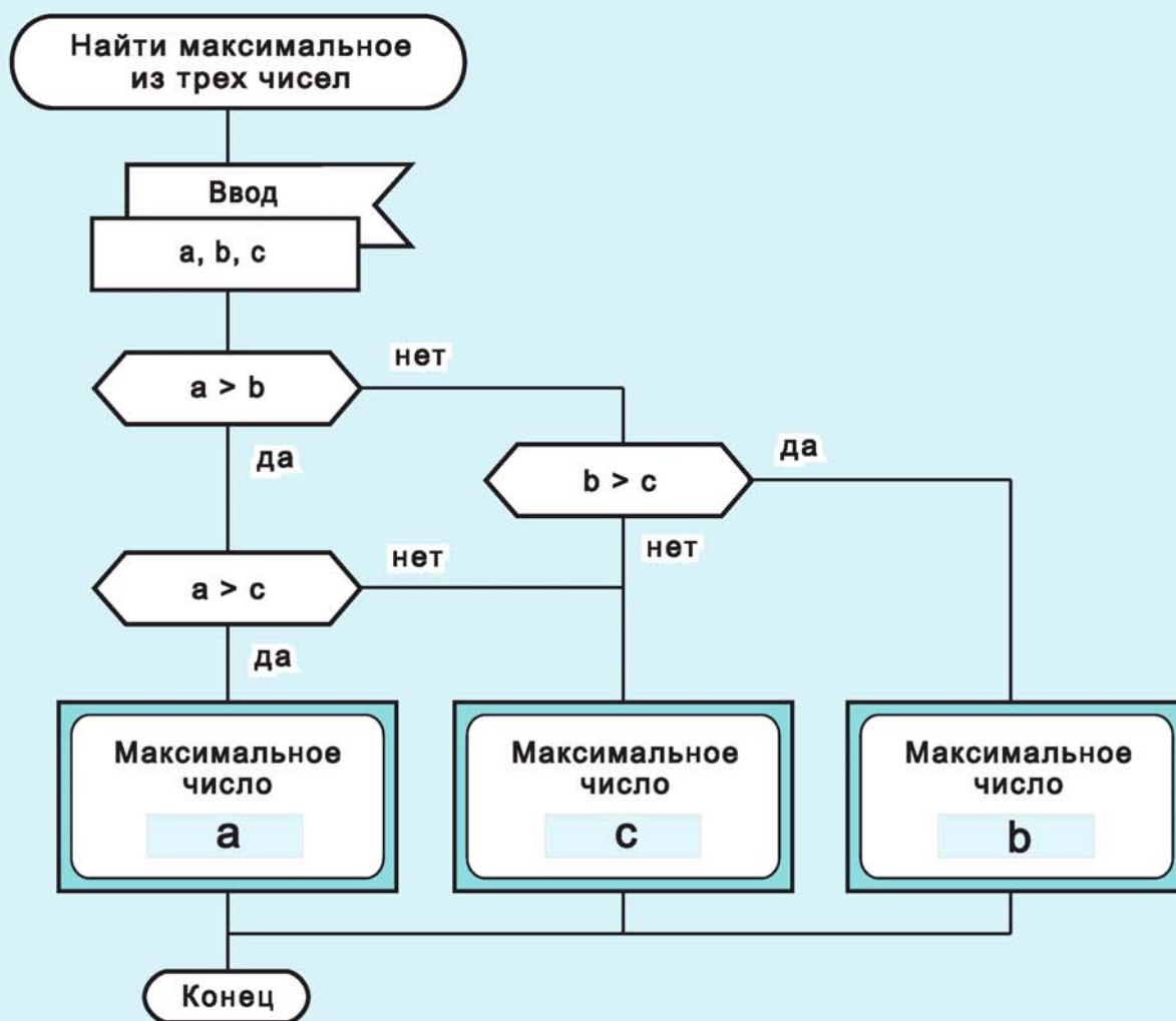
Рис. 210. Найти максимальное из трех чисел a, b, c
