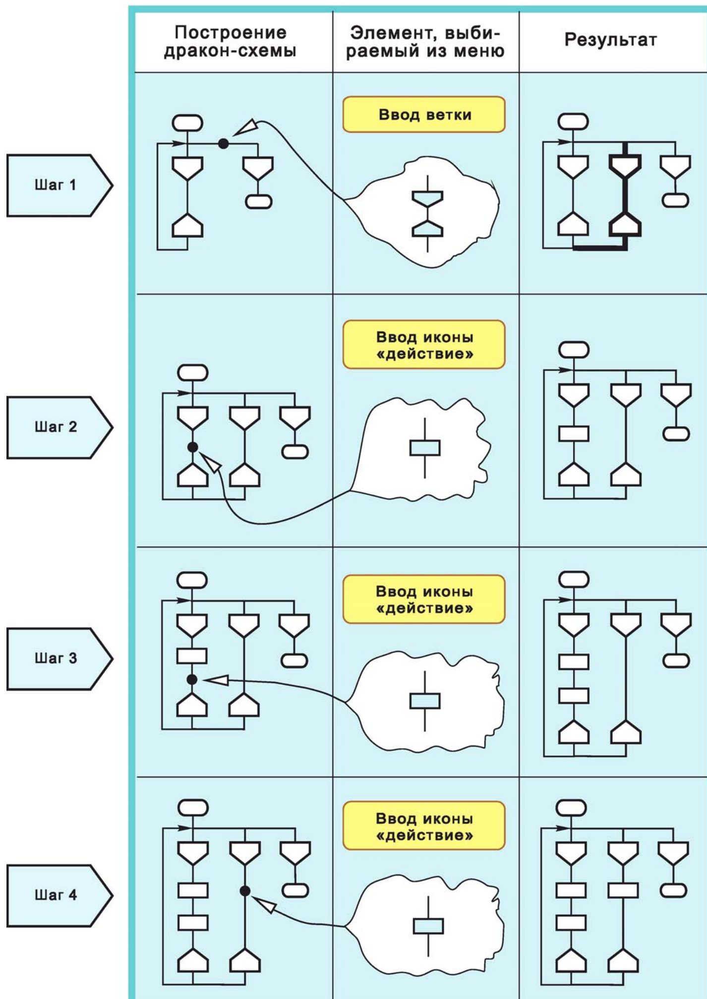
Рис. 239. Конструирование дракон-схемы «силуэт» с помощью дракон-конструктора
