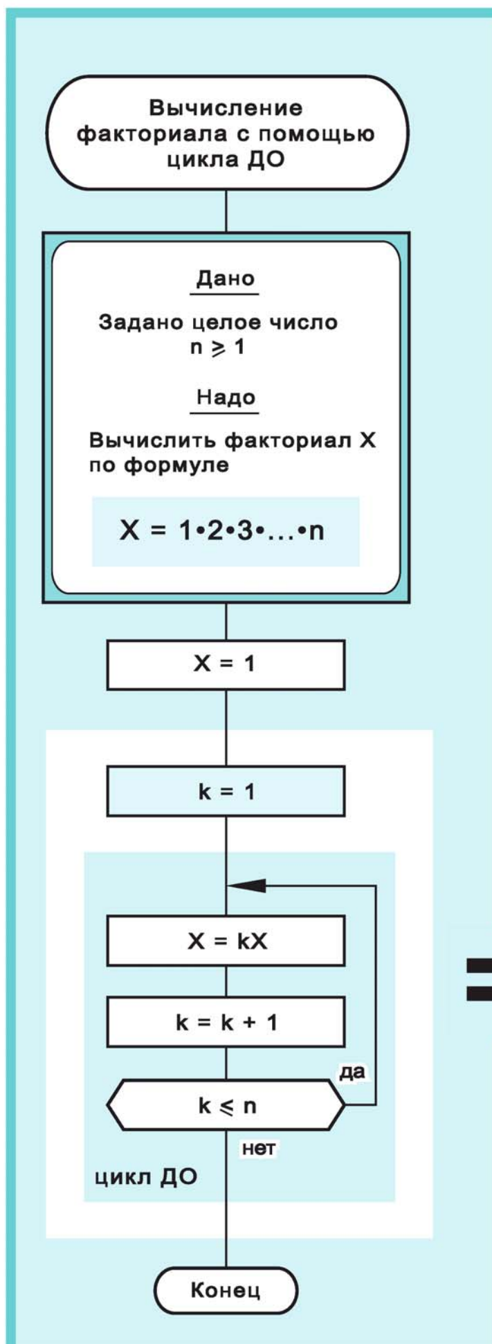
Рис. 90. Как вычислить факториал X = n! с помощью цикла ДО
