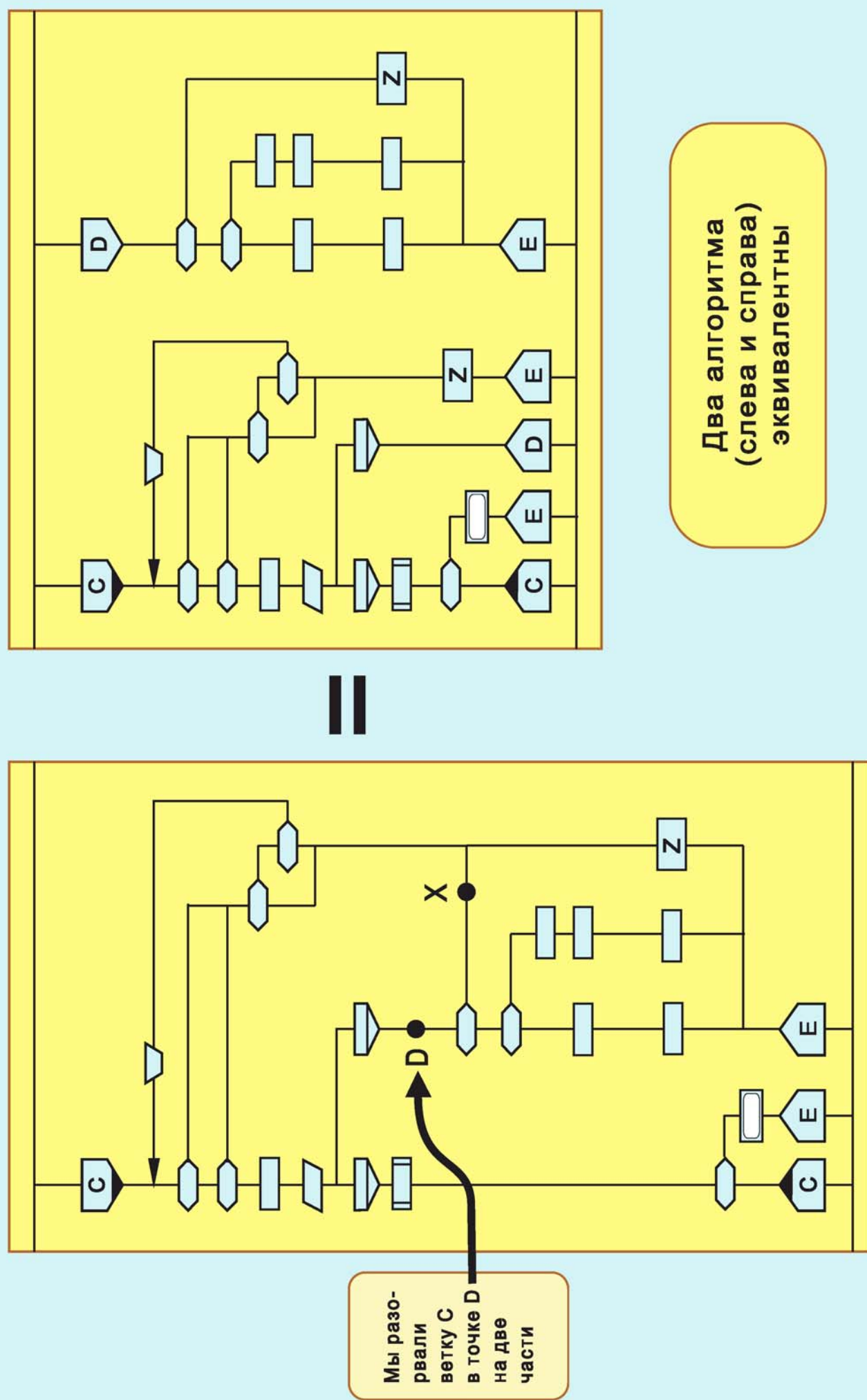
Рис. 228. Сложная ветка C (слева) превратилась в две простые ветки C и D (справа)
