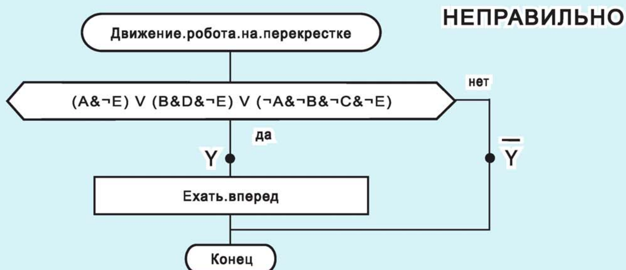
Рис. 133. Эргономически неудачная схема с абстрактными идентификаторами
