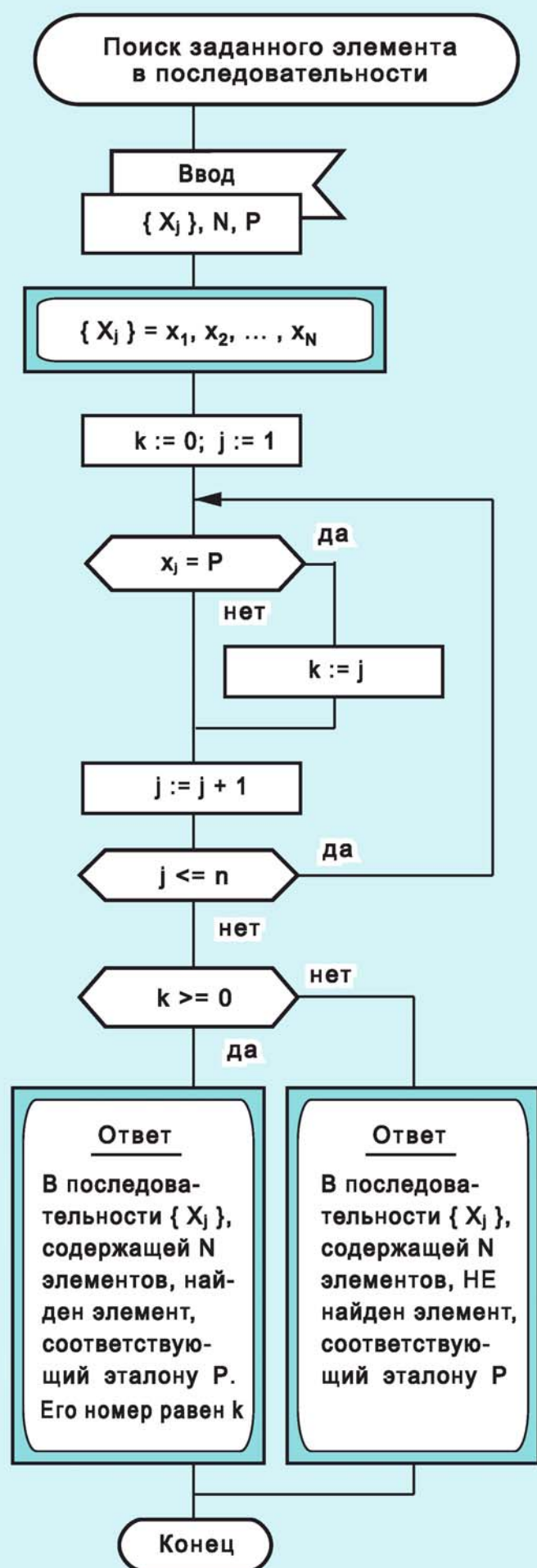
Рис. 214. Поиск заданного элемента в последовательности
