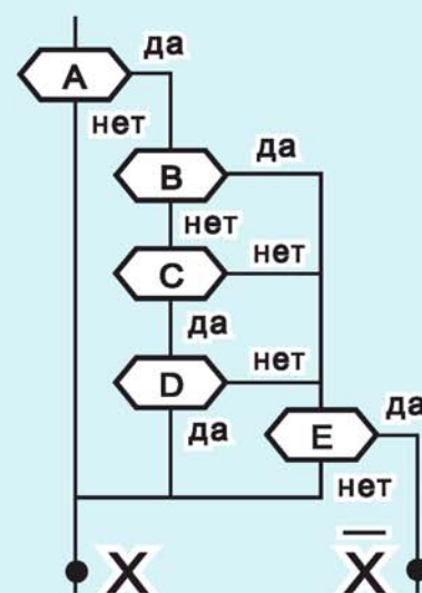
Рис. 125. Какую логическую функцию вычисляют эти схемы?
