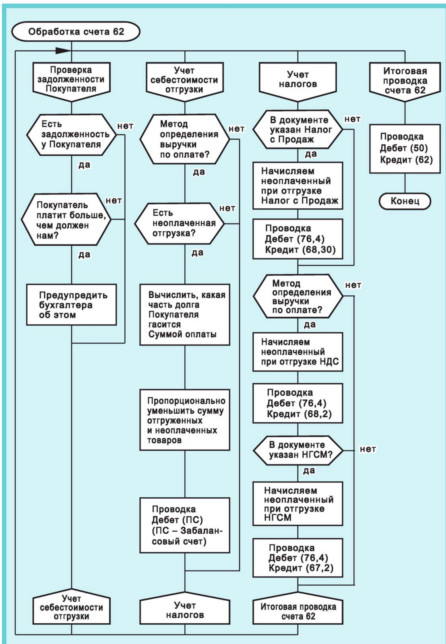
Рис. 181. Дракон-схема, описывающая обработку счета 62 при поступлении денег в кассу
