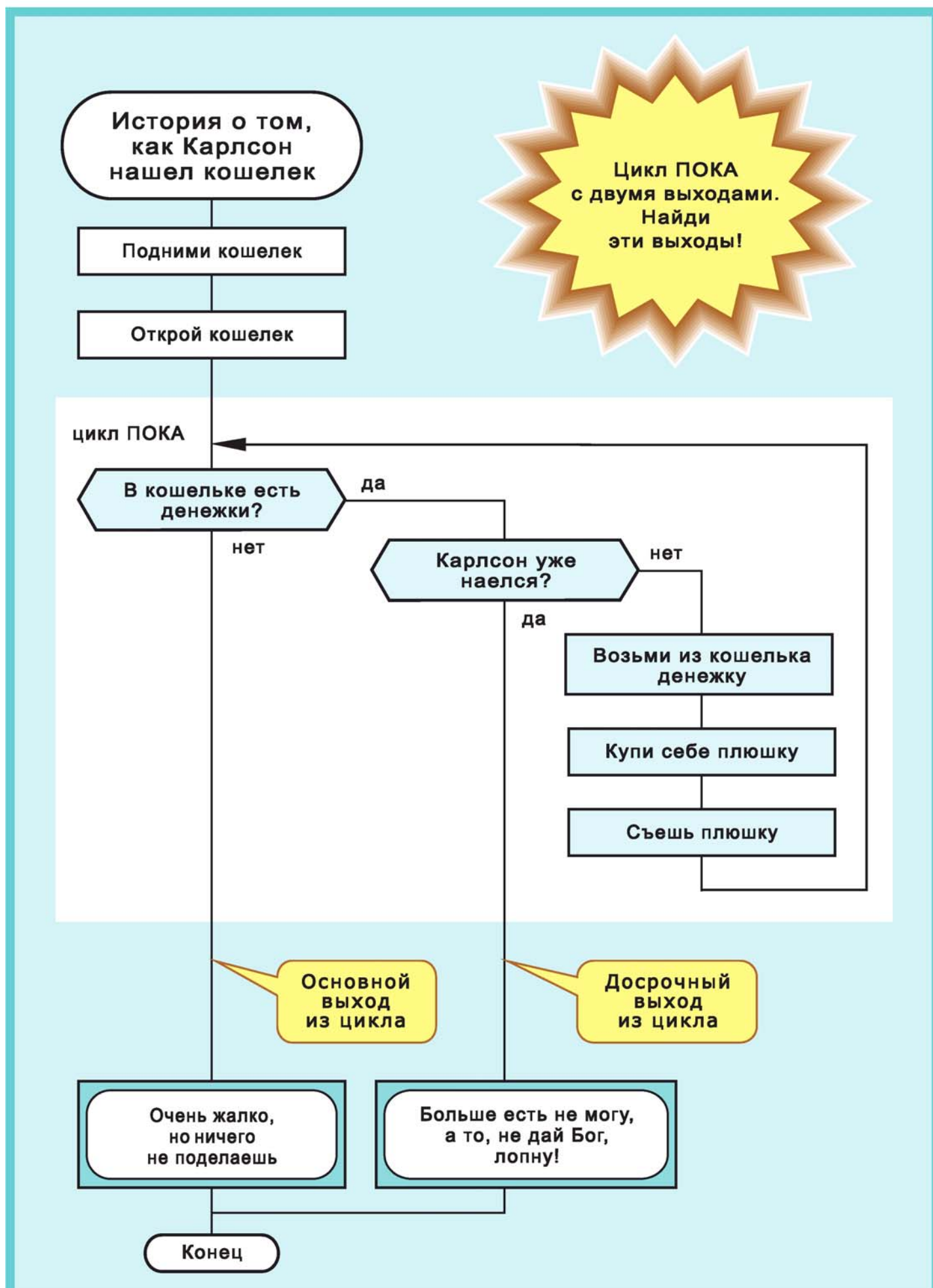
Рис. 81. Досрочный выход из цикла происходит потому, что Карлсон больше не хочет есть. Сравни с рис. 79
