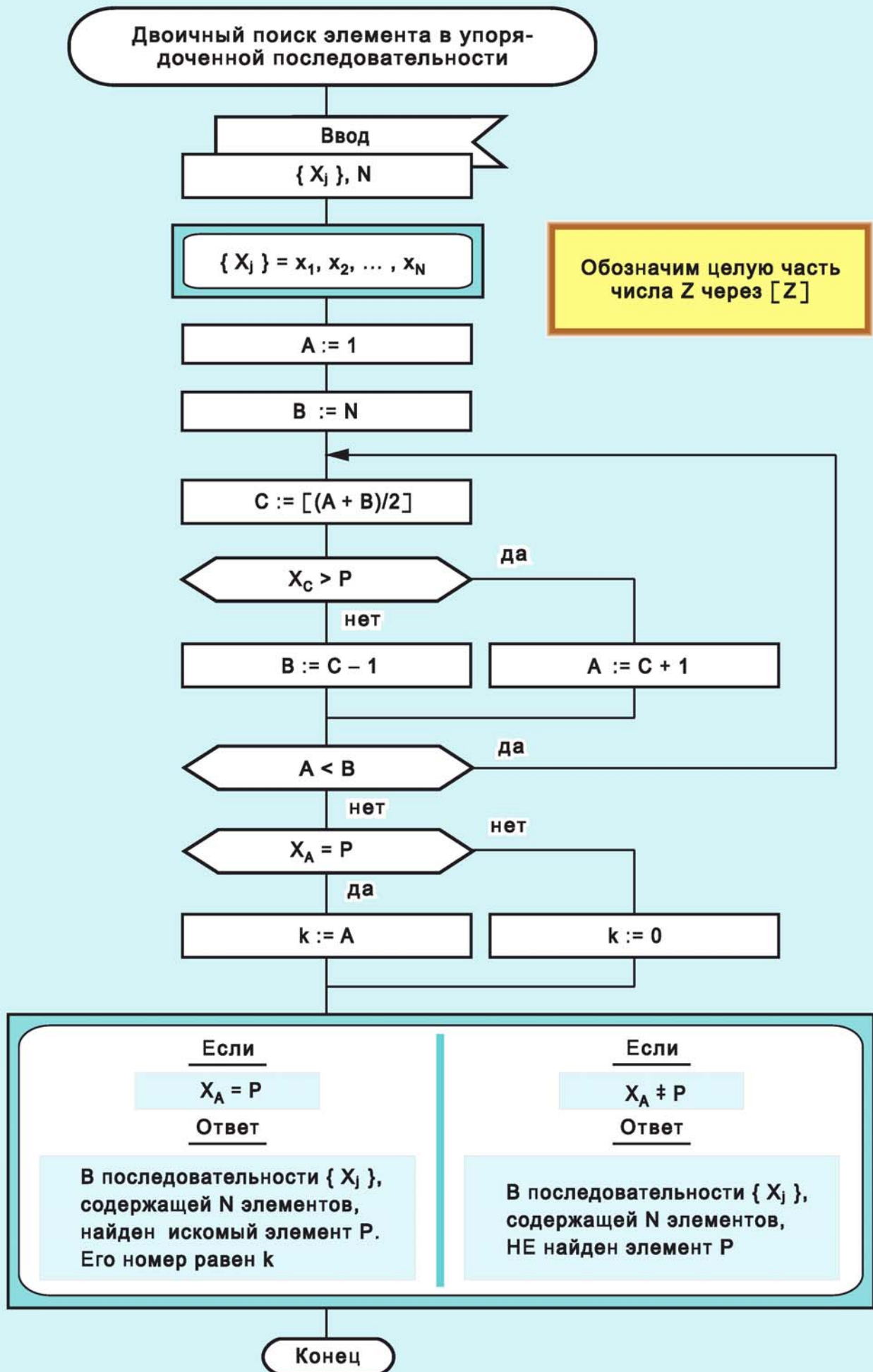
Рис. 216. Двоичный поиск элемента в упорядоченной последовательности
