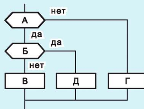
Рис. 64. Хорошая схема. Пересечение устранено
