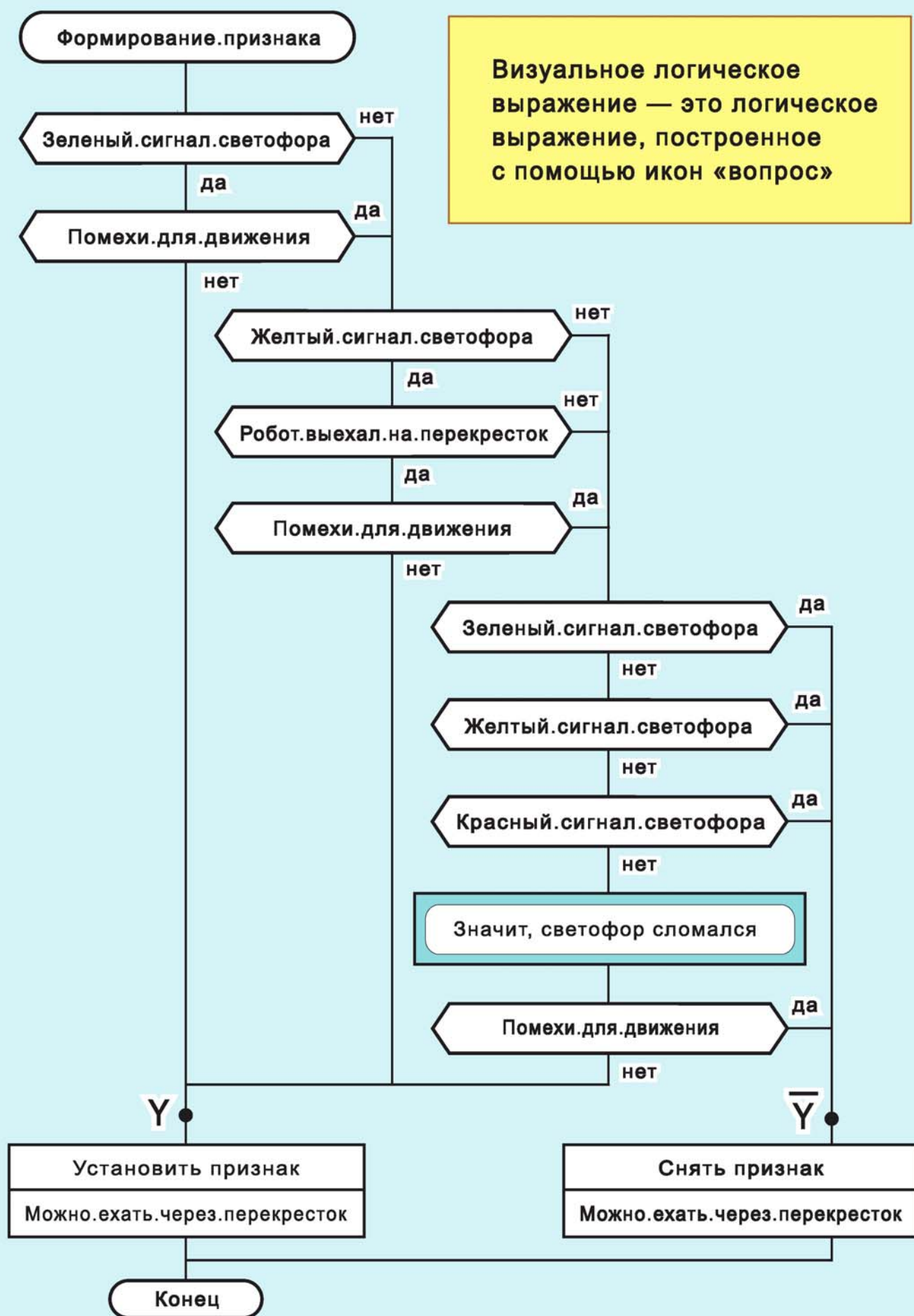
Рис. 138. Логический признак Y = \text{Можно.ехать.через.перекресток} вычисляется с помощью визуального логического выражения
