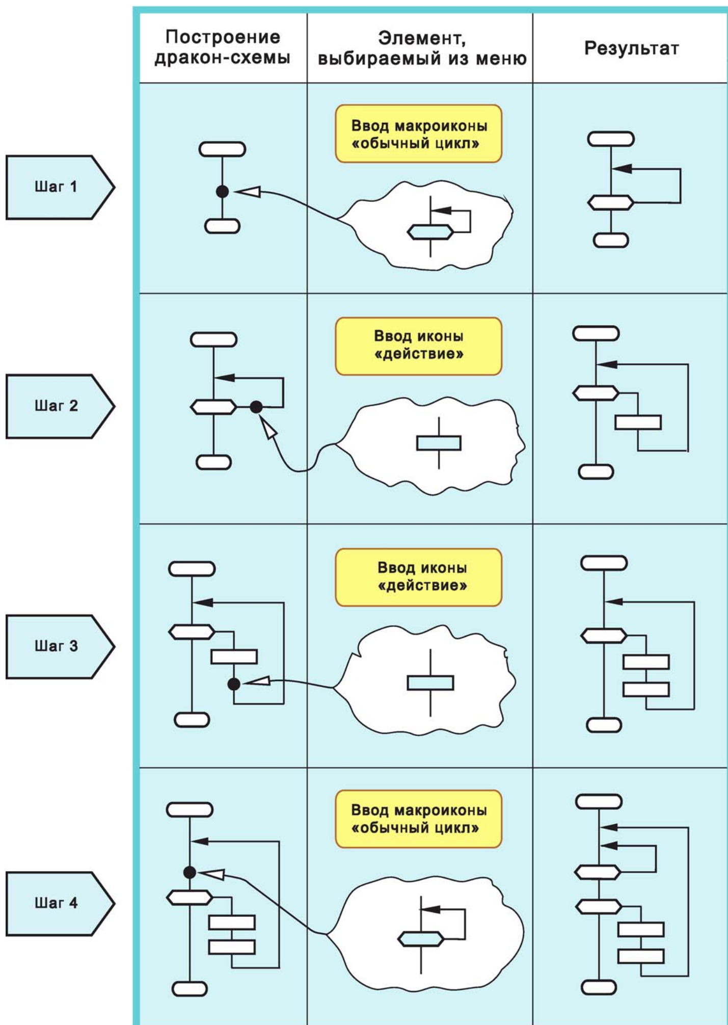
Рис. 234. Конструирование дракон-схемы «примитив» с помощью дракон-конструктора
