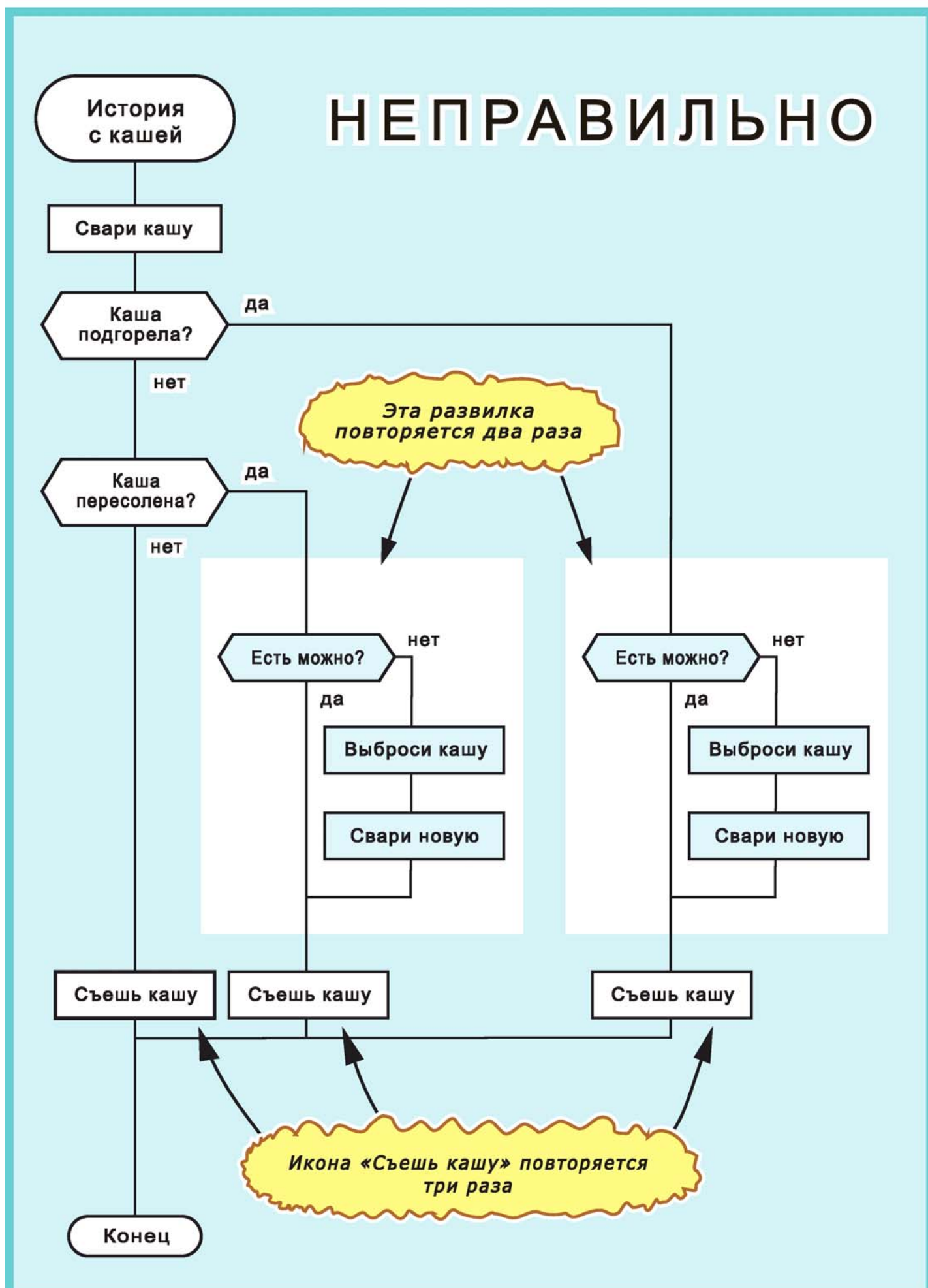
Рис. 54. Очень плохая дракон-схема. Правило «Повторы запрещены» нарушено в двух местах
