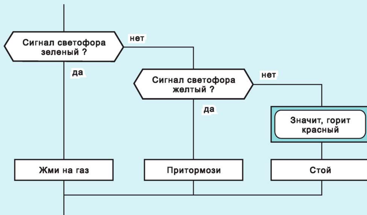
Рис. 13. Развилка на три направления, построенная с помощью иконы «Вопрос»
