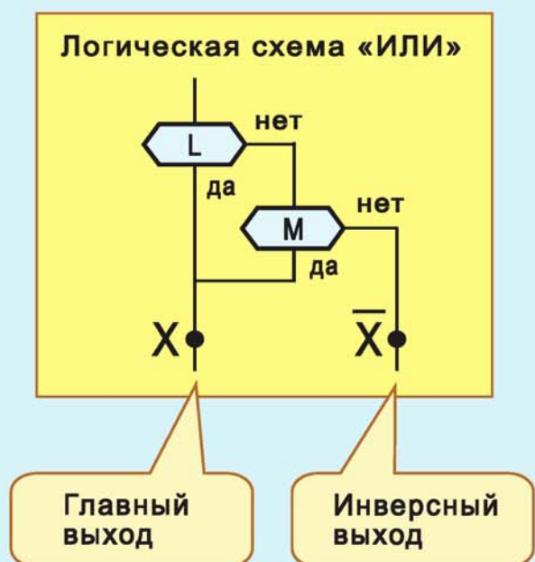
Рис. 116. Стандартный и нестандартный вид логической схемы «ИЛИ»
