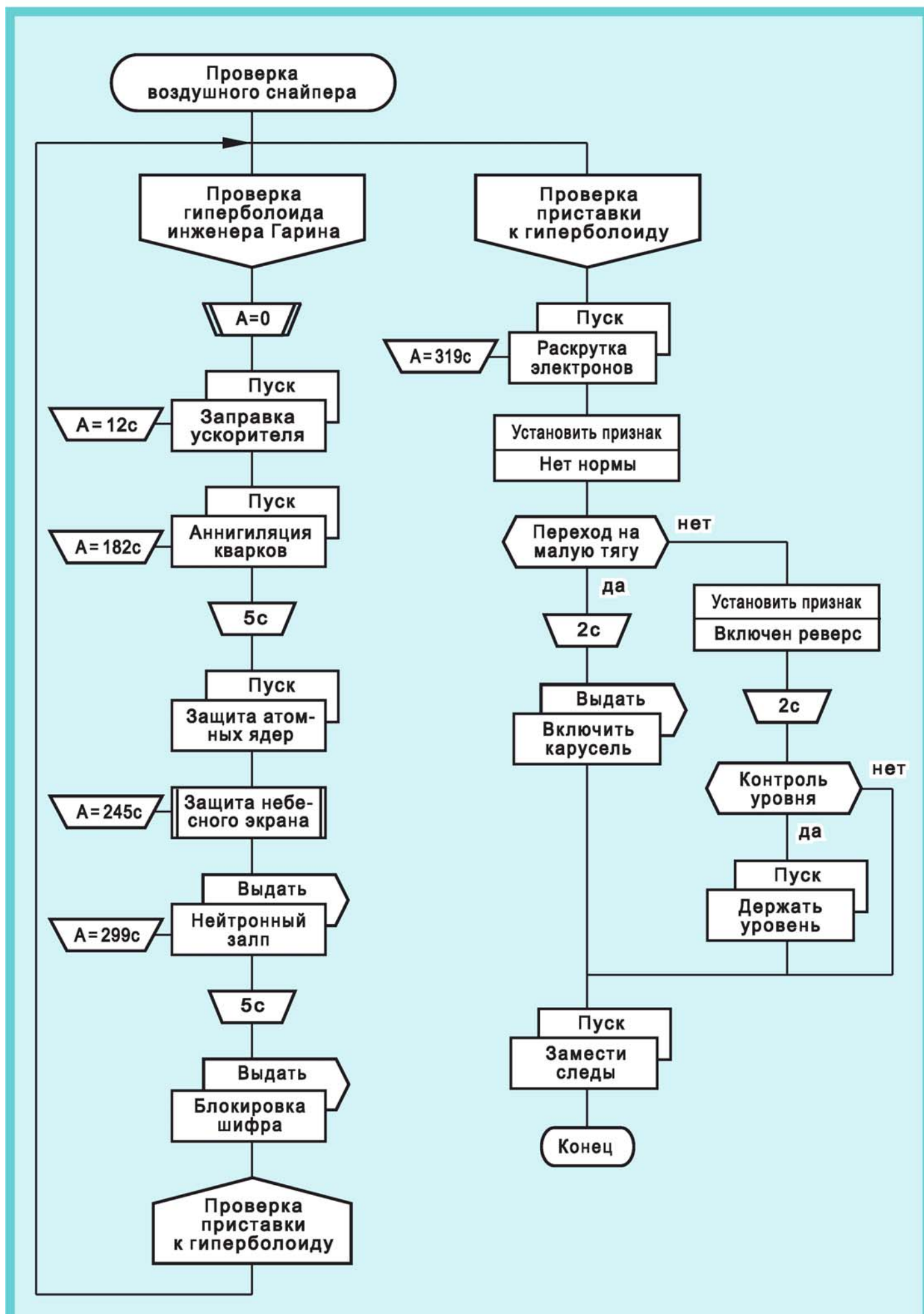
Рис. 151. Алгоритм с параллельными процессами «Проверка воздушного снайпера»
