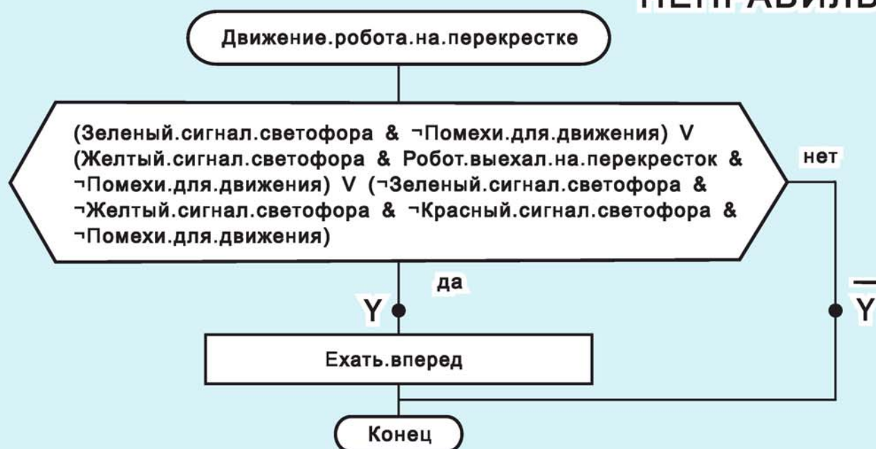
Рис. 135. Эргономически неудачная схема. Несмотря на замену коротких смысловых идентификаторов на длинные и понятные, текст в иконе «вопрос» все еще очень труден.
