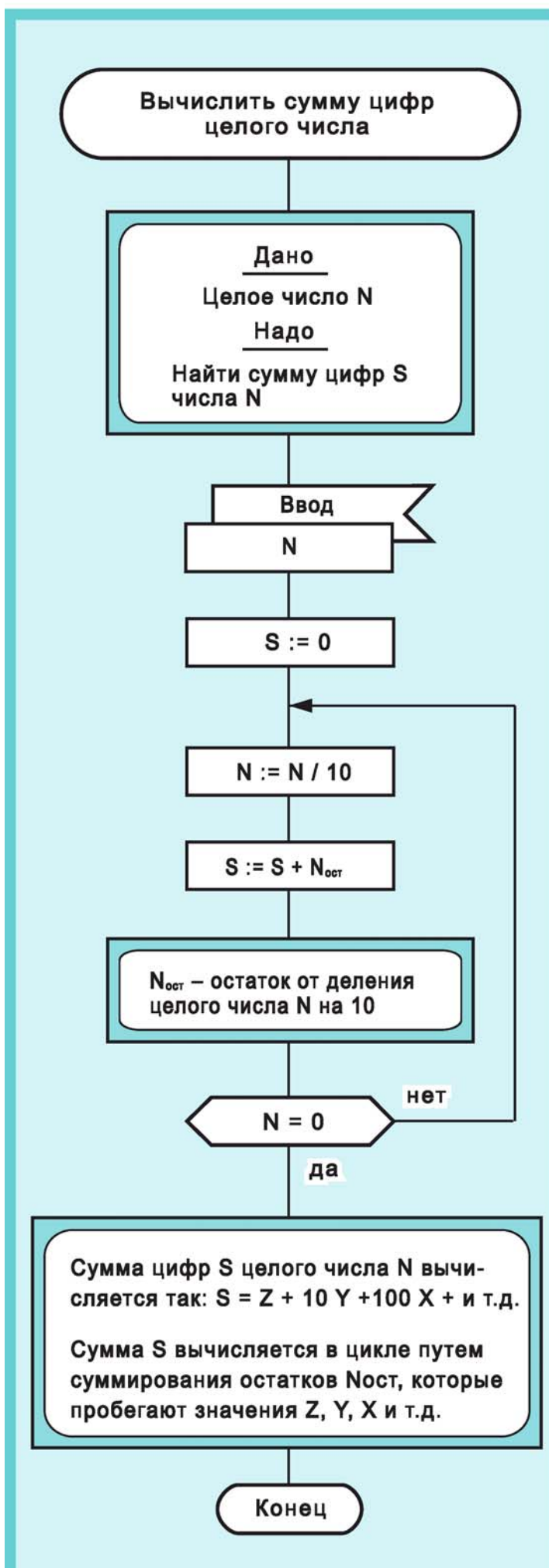
Рис. 208. Вычислить сумму цифр целого числа
