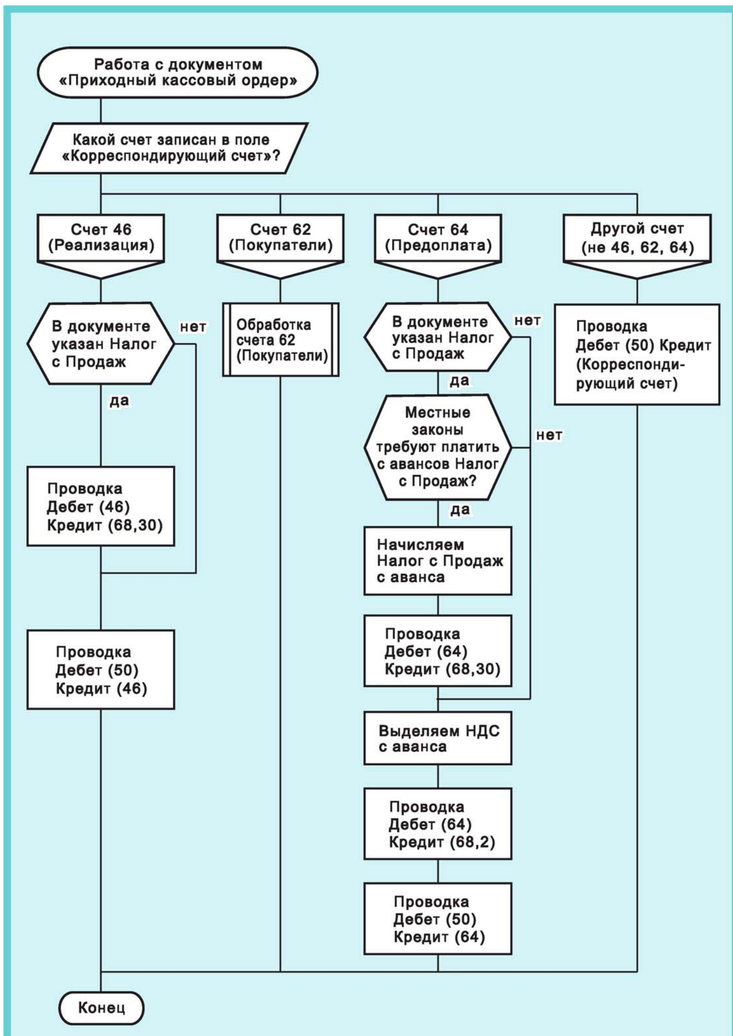
Рис. 179. Дракон-схема, описывающая работу с документом «Приходный кассовый ордер»
