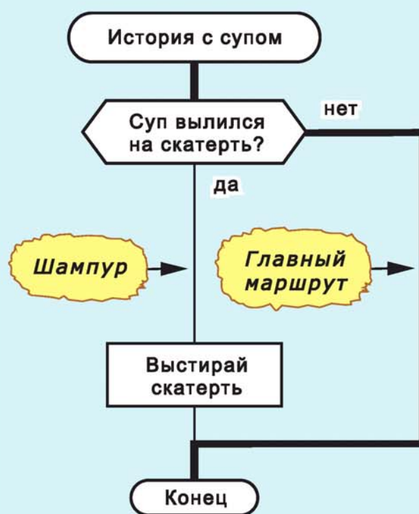
Рис. 30. Плохая схема. Нарушено правило «Главный маршрут должен идти по шампуру»
