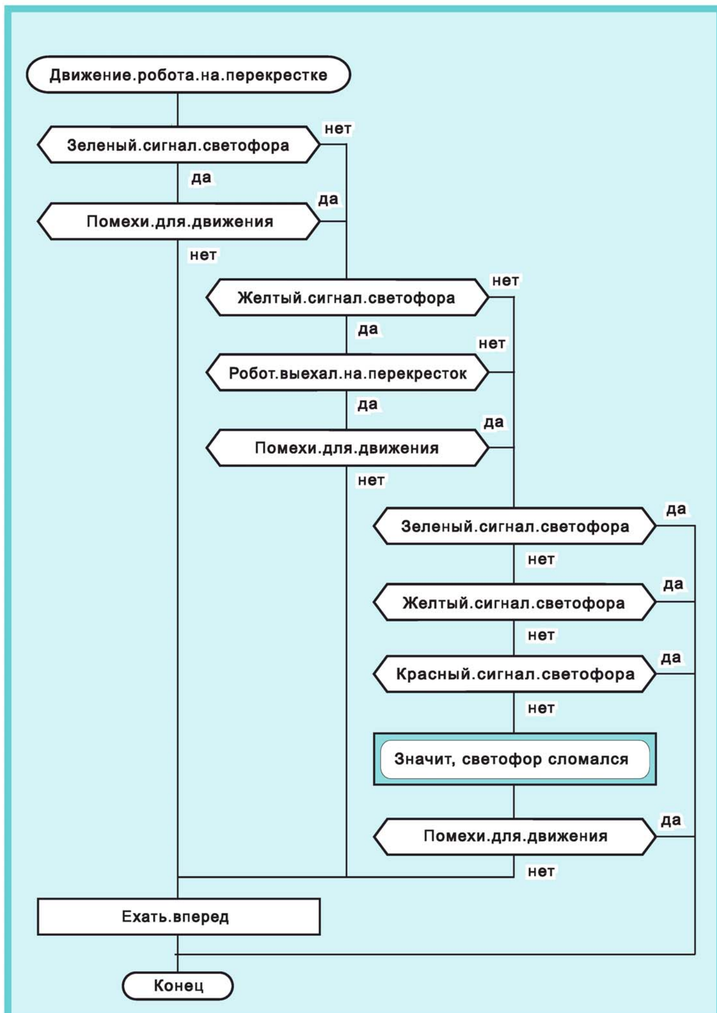
Рис. 128. Алгоритм «Движение робота на перекрестке»
