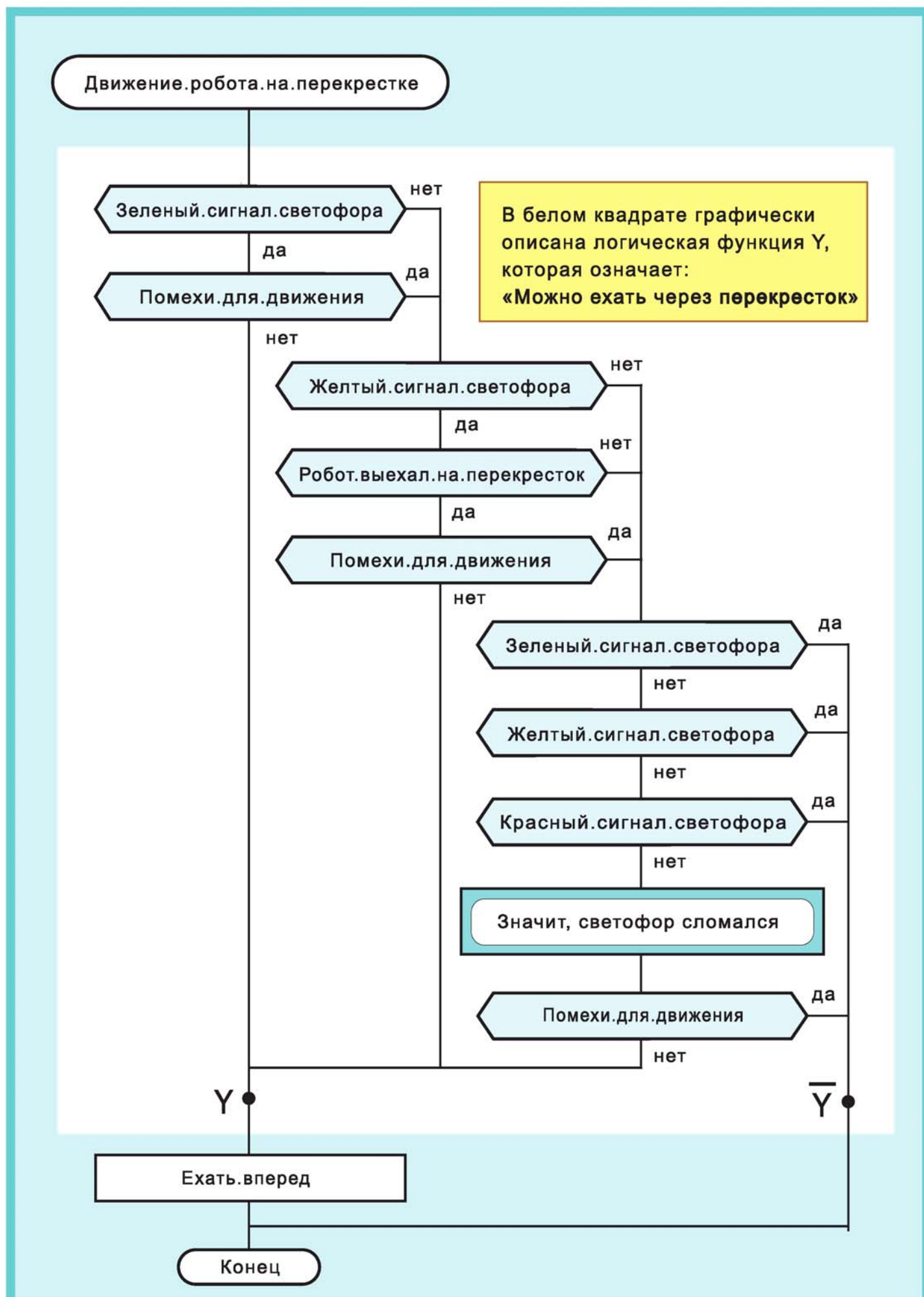
Рис. 129. Выделена логическая функция Y «Можно ехать через перекресток»
