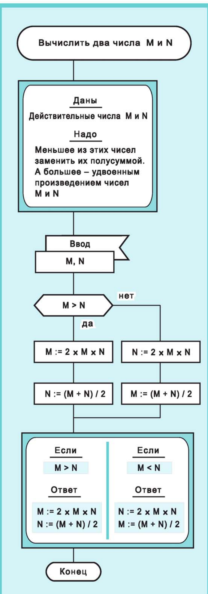
Рис. 209. Вычислить два числа M и N
