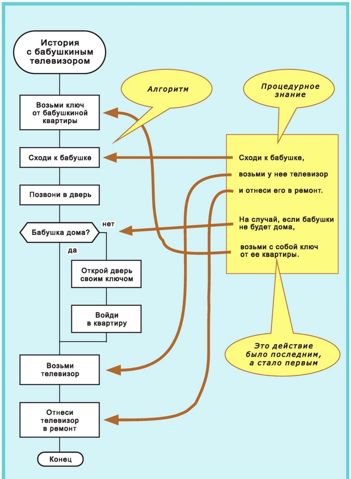
Рис. 11. Чтобы превратить процедурное знание в алгоритм, иногда приходится изменять порядок действий (см. стрелки)
