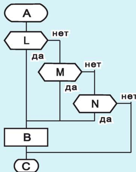
Рис. 112. Математическая формула и дракон-схема «ИЛИ»
