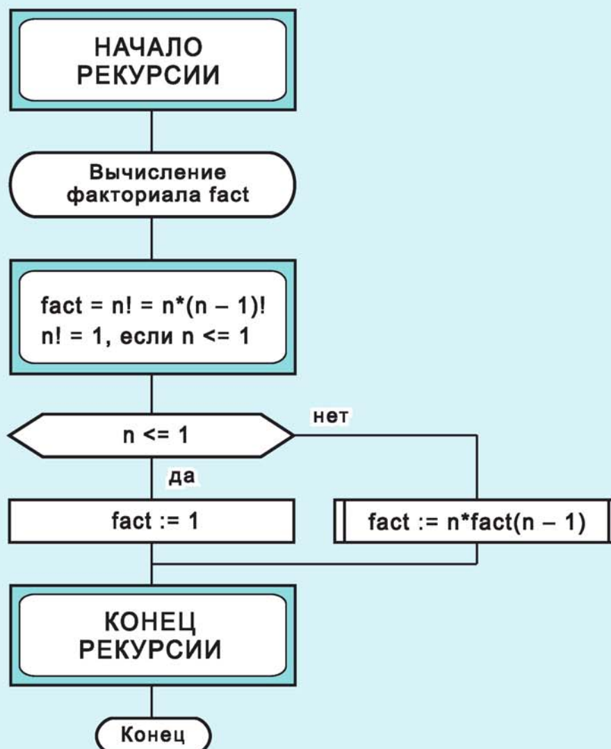
Рис. 217. Рекурсивная функция «Вычисление факториала fact»
