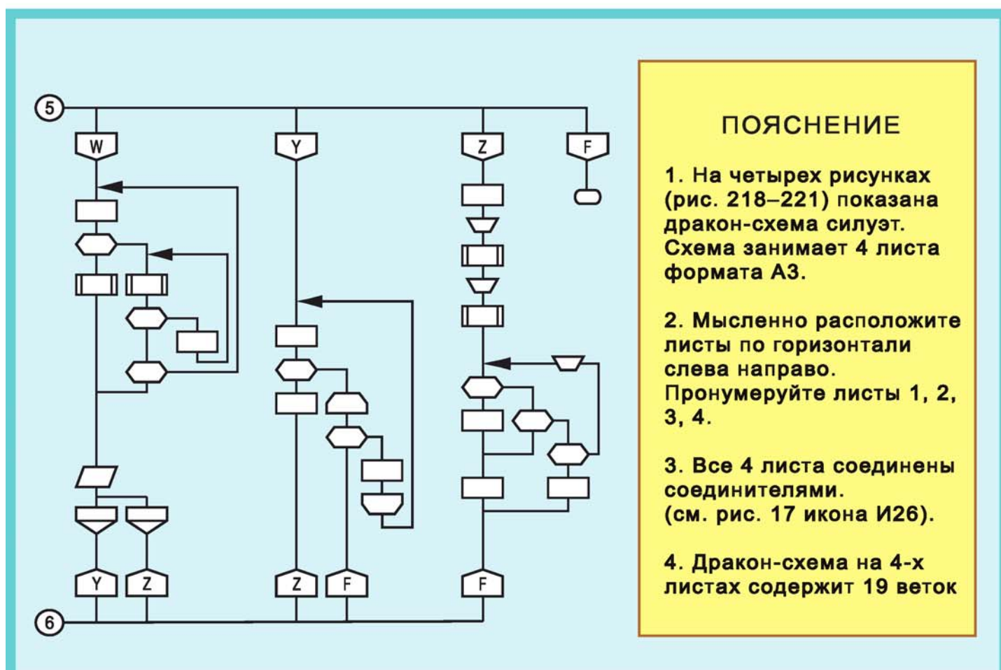
Рис. 221. Лист 4. (Комплект из 4-х листов формата А3)
