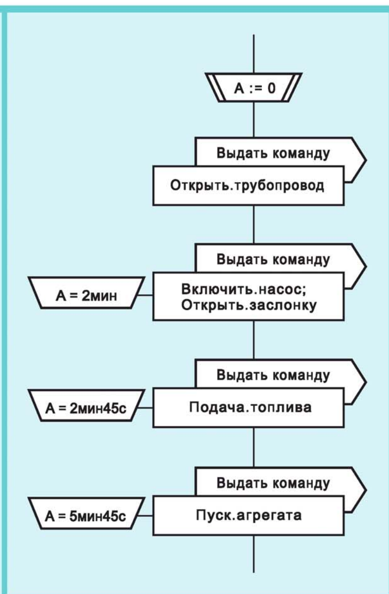
Рис. 143. Пример использования операторов «пуск таймера» и «синхронизатор»
