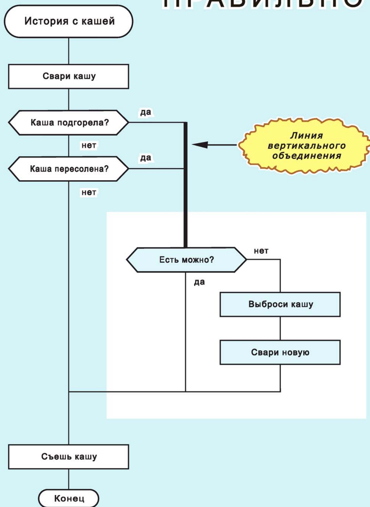
Рис. 56. Хорошая (ясная и наглядная) дракон-схема. Все повторы устранены. Данная схема получена из рис. 55 в результате объединения двух развилок «Есть можно?»
