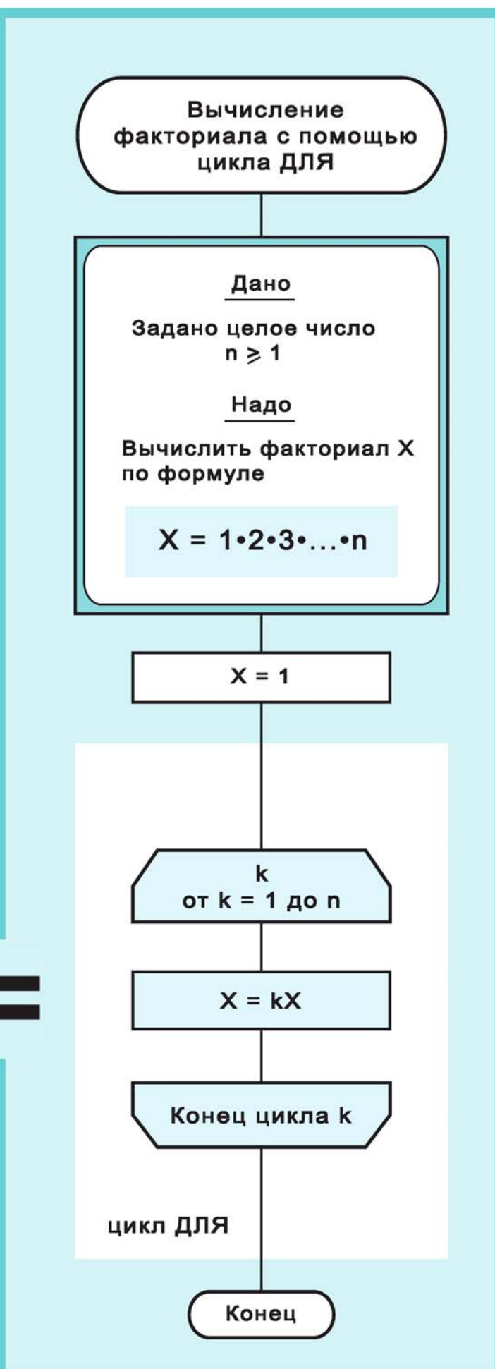
Рис. 91. Как вычислить факториал X = n! с помощью цикла ДЛЯ
