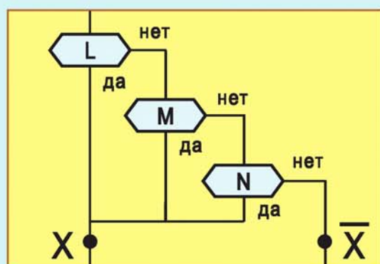
Рис. 122. Стандартный и нестандартный вид логических схем «И», «ИЛИ» для трех логических переменных
