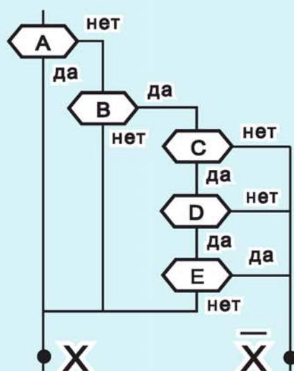
Рис. 125. Какую логическую функцию вычисляют эти схемы?
