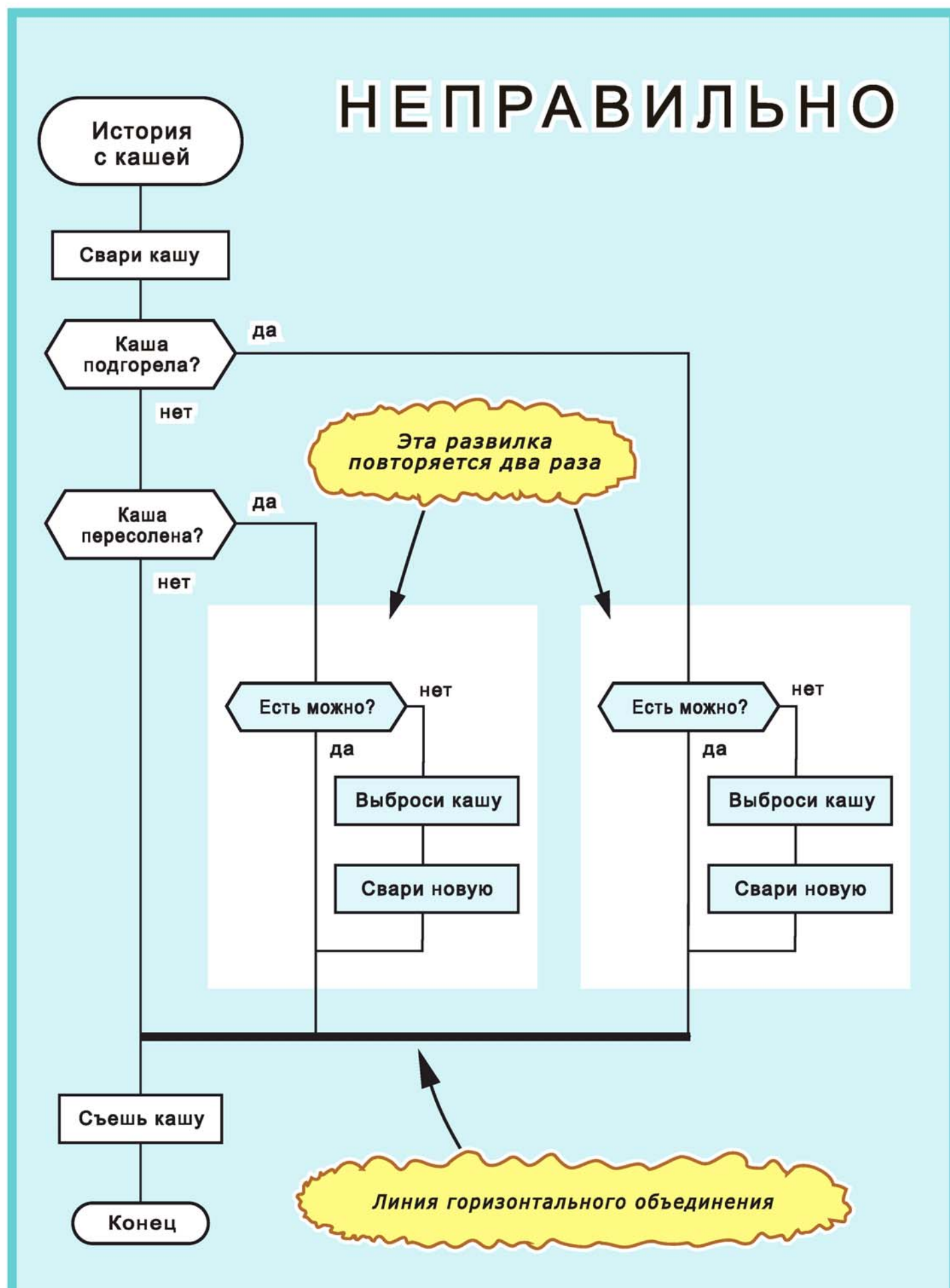
Рис. 55. Данная схема получена из рис. 54 в результате объединения трех икон «Съешь кашу». Однако работа еще не закончена. Нужно устранить оставшиеся повторы
