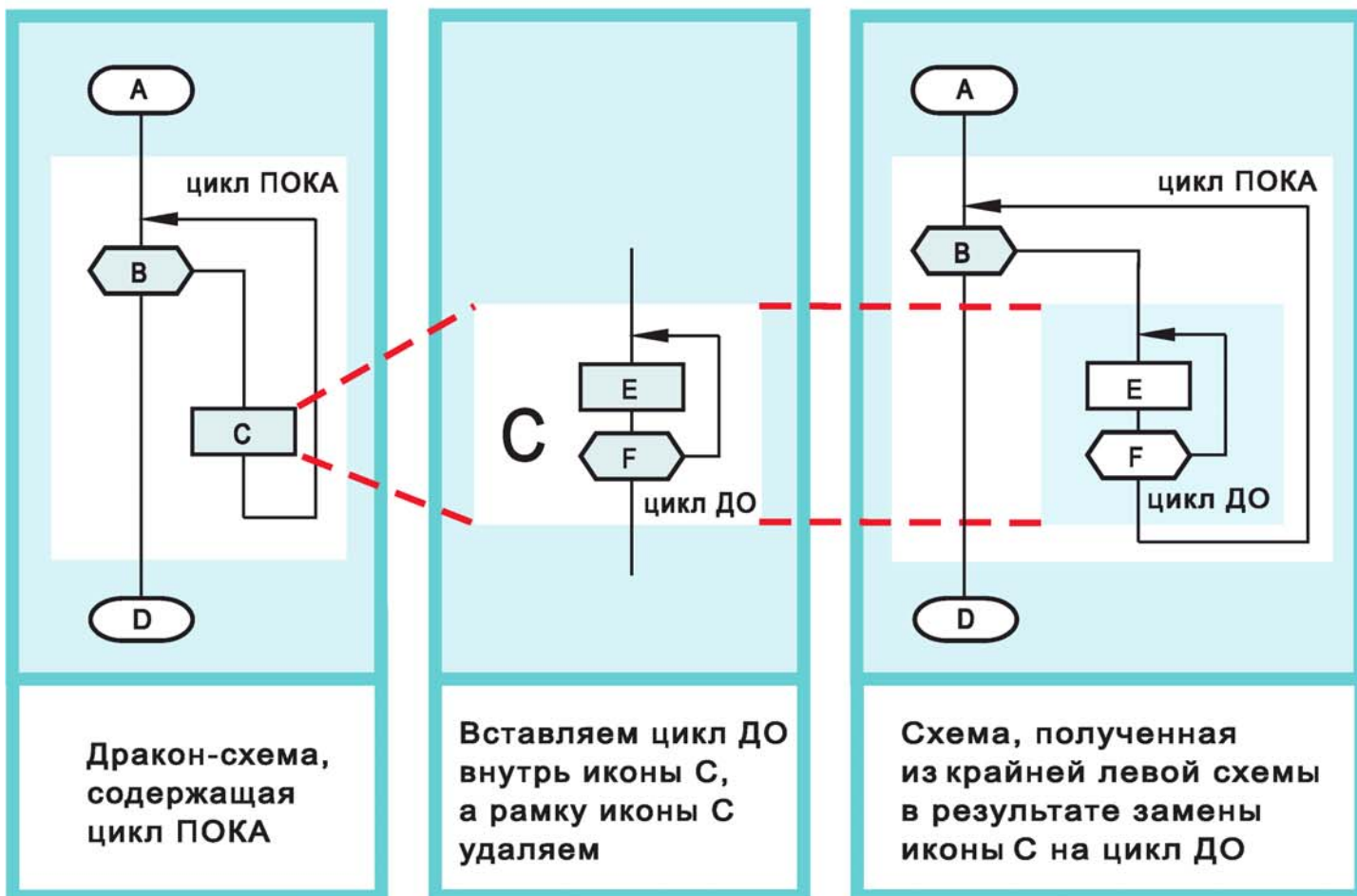
Рис. 99. Как построить цикл в цикле
