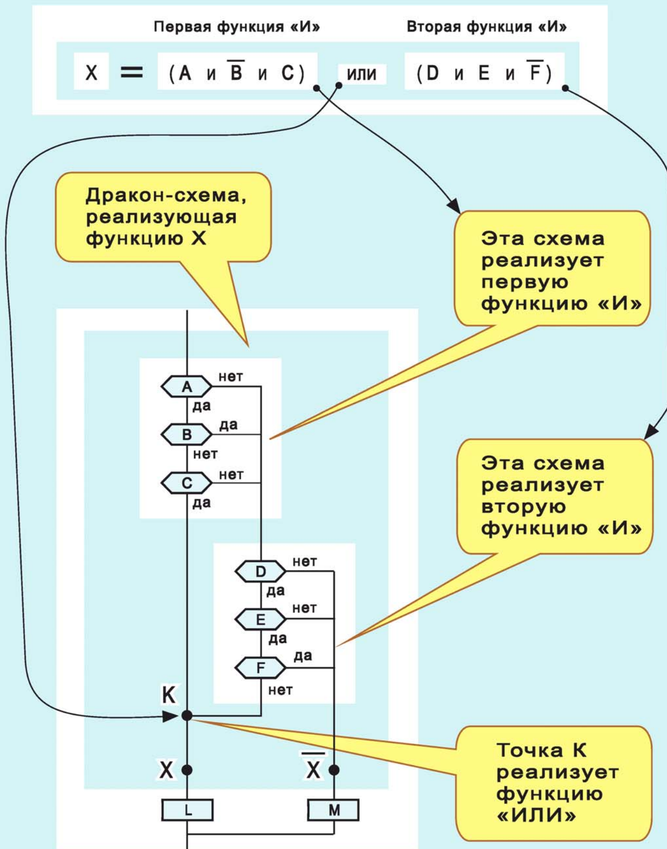
Рис. 123. Как нарисовать дракон-схему для сложной логической функции?
