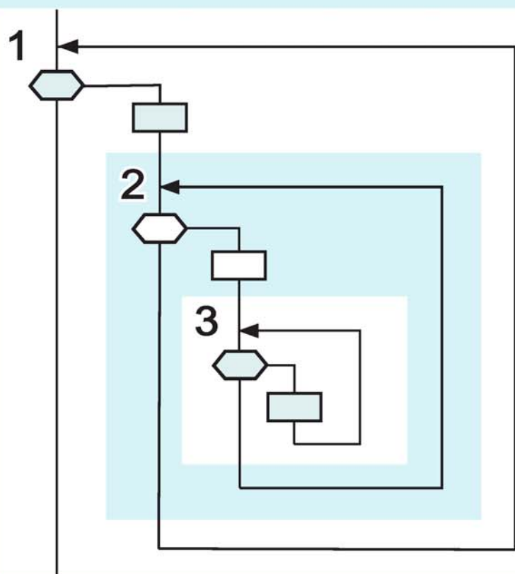
Рис. 102. Цикл ПОКА (3) внутри цикла ПОКА (2) внутри цикла ПОКА (1)
