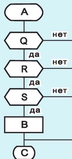
Рис. 107. Математическая формула и дракон-схема «И»
