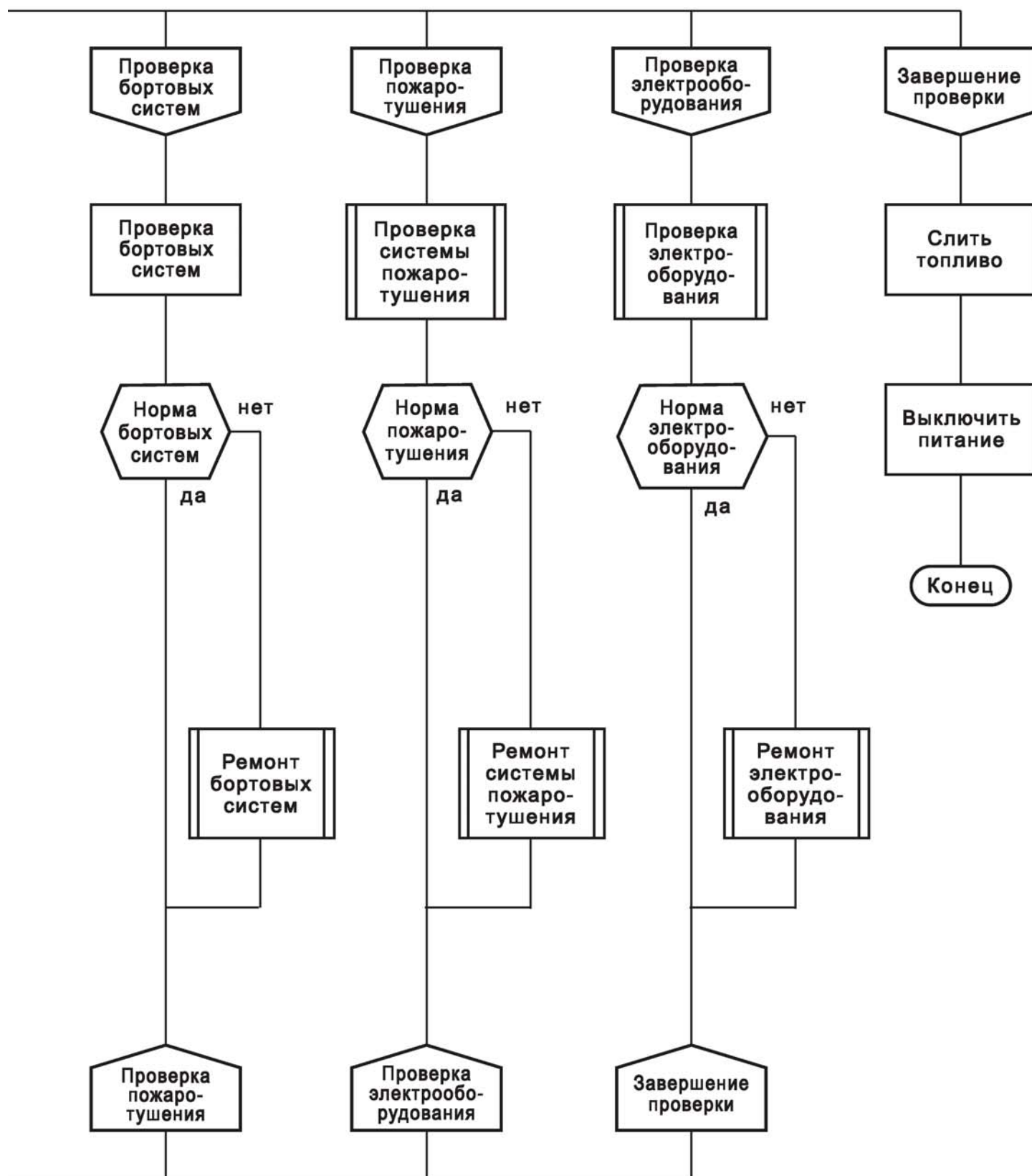
Рис. 172. Алгоритм «Проверка самолета»
